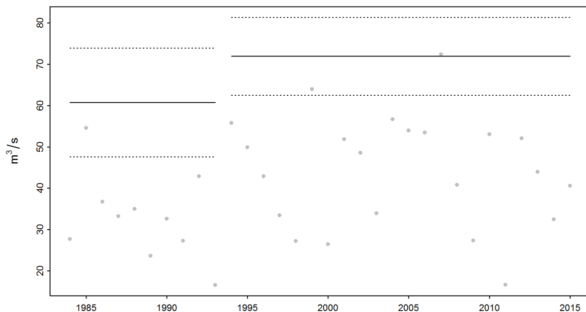
FIGURE 7 – Modification des HQ 100 (calculés à l'aide de la variante «mujump1994») et de l'intervalle de confiance à 95 % (méthode delta ; lignes en traitillé) durant la période 1984-2015
