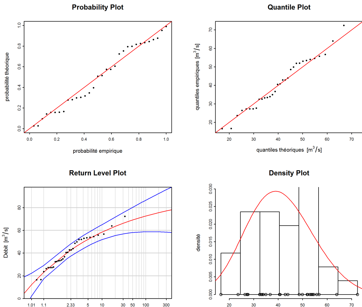
FIGURE 5 – Graphiques diagnostiques de la variante «stat» de la méthode BLOCK(1984-2015)
