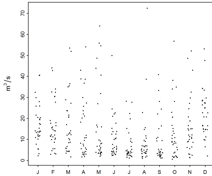
FIGURE 3 – Variations saisonnières des maxima mensuels [ \text{m}^3/\text{s} ] (01.01.1984 - 31.12.2015)
