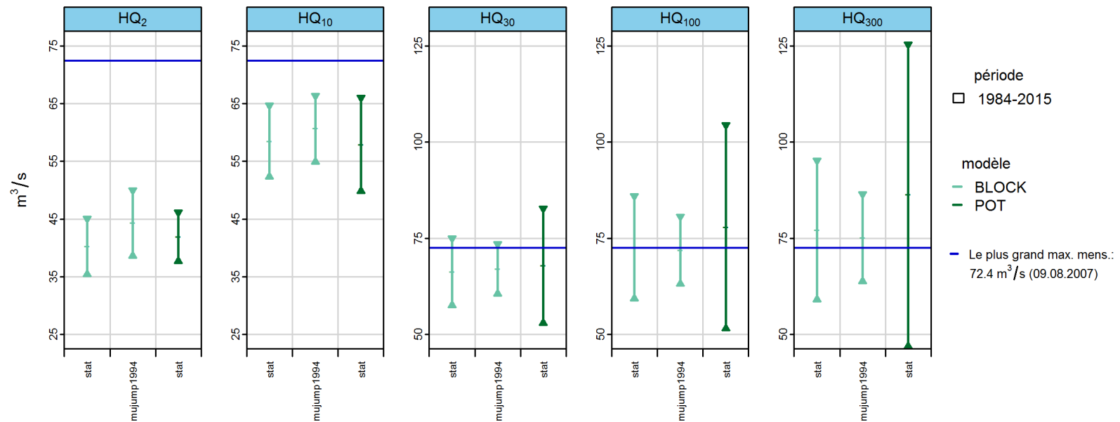
FIGURE 10 – HQ T [m³/s] y c. un intervalle de confiance à 95 % calculé à l'aide du modèle stationnaire ainsi qu'au moyen de la meilleure variante de la méthode BLOCK et POT pour l'année 2015
