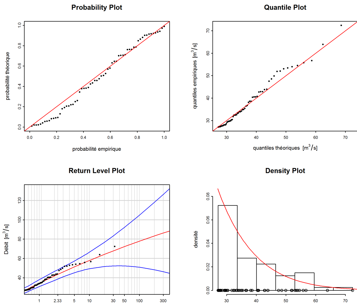
FIGURE 9 – Graphiques diagnostiques de la variante «stat» de la méthode POT (1984-2015)
