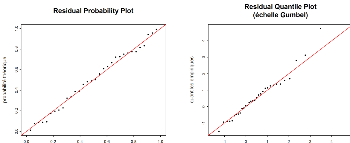
FIGURE 6 – Graphiques diagnostiques de la variante «mujump1994» de la méthode BLOCK (1984-2015)
