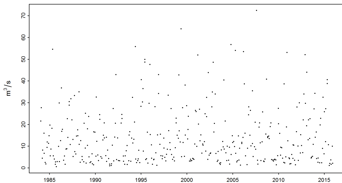
FIGURE 2 – Série chronologique des maxima mensuels [ \text{m}^3/\text{s} ] (01.01.1984 - 31.12.2015)
