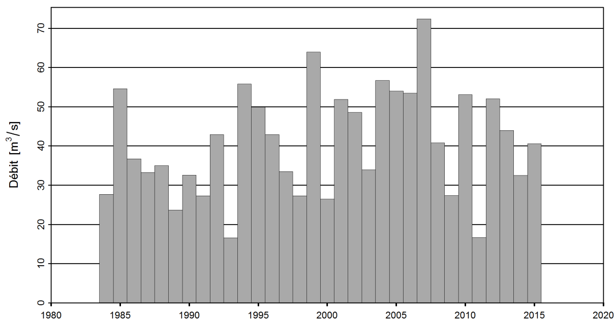
FIGURE 1 – Série chronologique des maxima annuels [ \text{m}^3/\text{s} ] (1984 - 2015, gris foncé : maxima annuels pris en compte)
