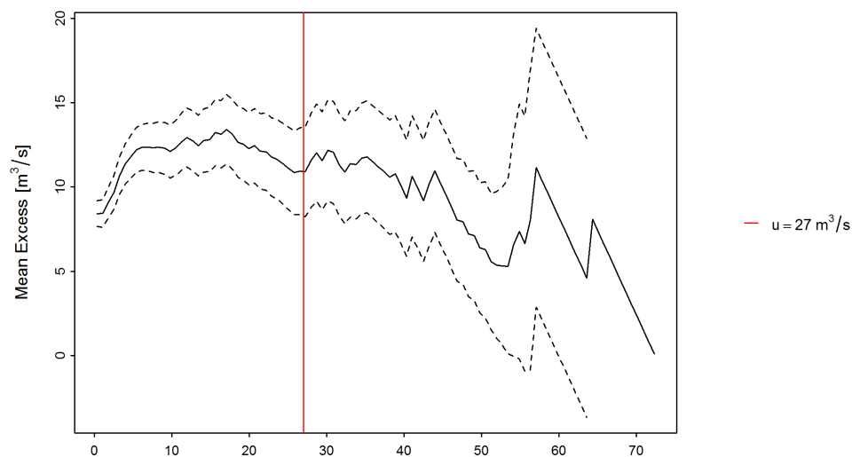
FIGURE 11 – «mean residual life plot» avec le seuil déterminé u (ligne rouge), dépassement moyen (ligne noire), intervalle de confiance à 95 % (traitillés)
