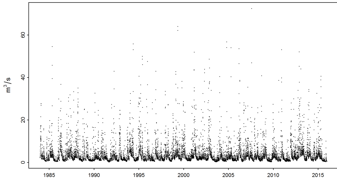
FIGURE 4 – Série chronologique des maxima journaliers [ \text{m}^3/\text{s} ] (01.01.1984 - 31.12.2015)
