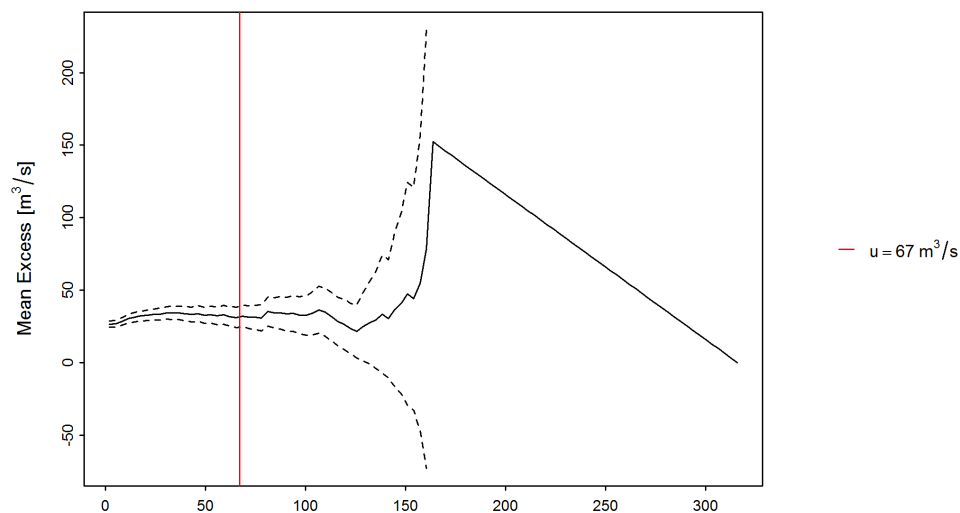
FIGURE 9 – «mean residual life plot» avec le seuil déterminé u (ligne rouge), dépassement moyen (ligne noire), intervalle de confiance à 95 % (traitillés)
