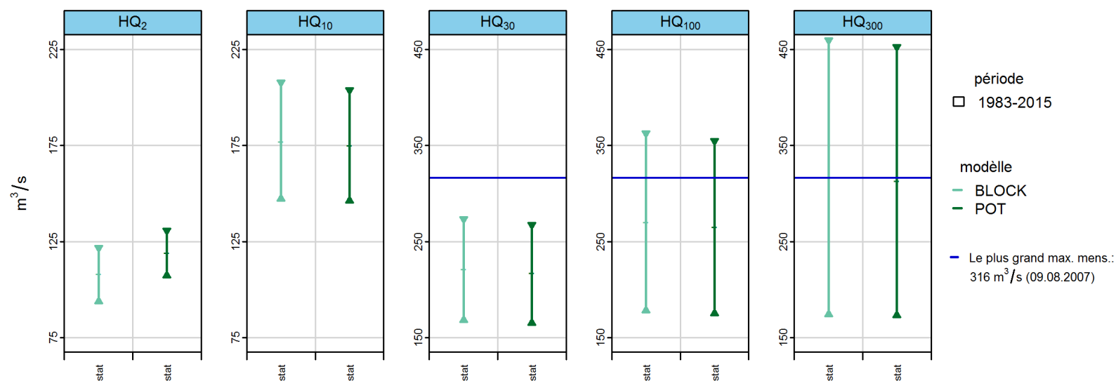
FIGURE 8 – HQ T [m³/s] y c. un intervalle de confiance à 95 % calculé à l'aide du modèle stationnaire ainsi qu'au moyen de la meilleure variante de la méthode BLOCK et POT pour l'année 2015
