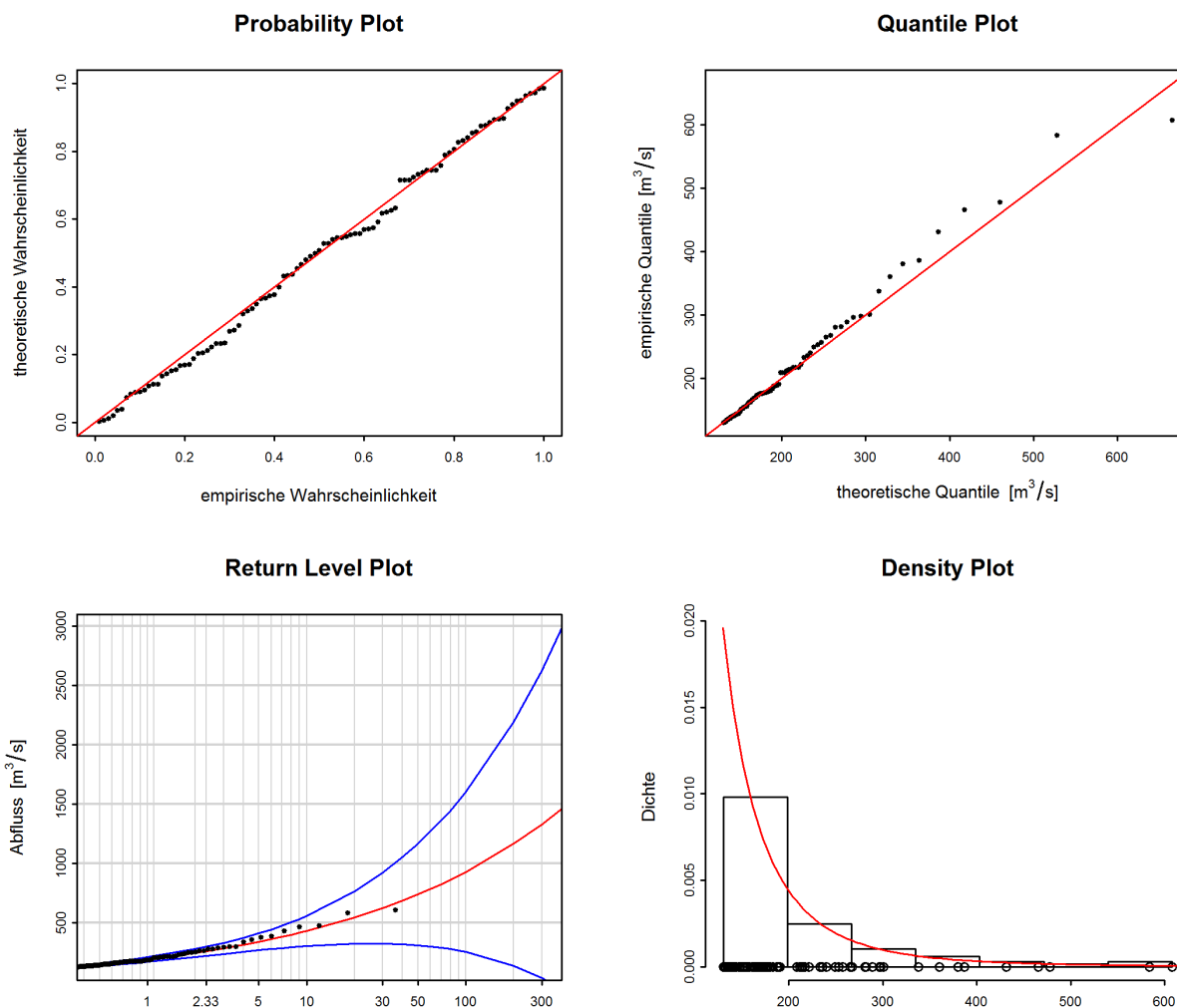
Abbildung 7: Diagnostikplots der Modellvariante „stat“ des POT-Ansatzes (1980-2015)
