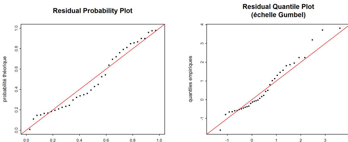
FIGURE 6 – Graphiques diagnostiques de la variante «mujump1992» de la méthode BLOCK (1980-2015)
