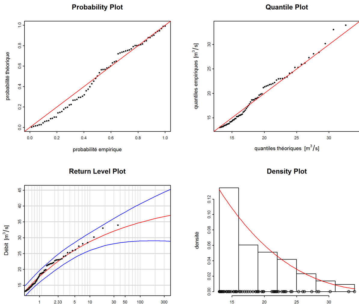
FIGURE 9 – Graphiques diagnostiques de la variante «stat» de la méthode POT (1980-2015)
