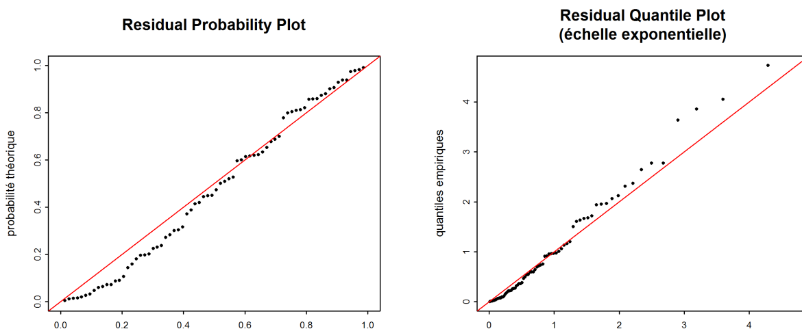
FIGURE 10 – Graphiques diagnostiques de la variante «sigjump1992» de la méthode POT (1980-2015)
