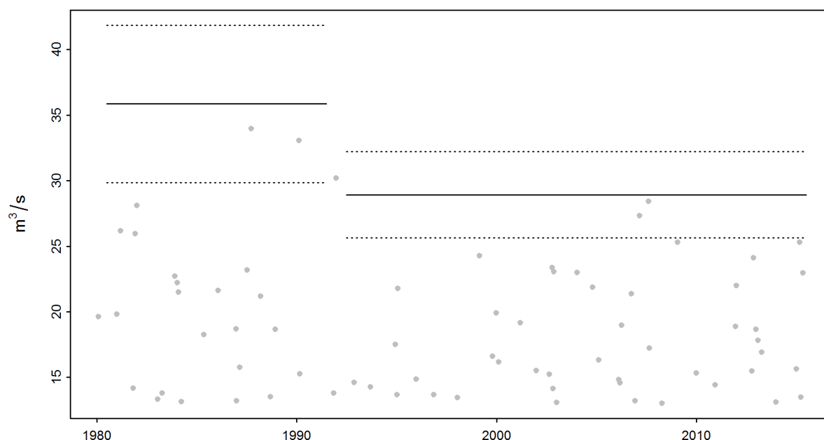
FIGURE 11 – Modification des HQ 100 (calculés à l'aide de la variante «sigjump1992») et de l'intervalle de confiance à 95 % (méthode delta ; lignes en traitillé) durant la période 1980-2015
