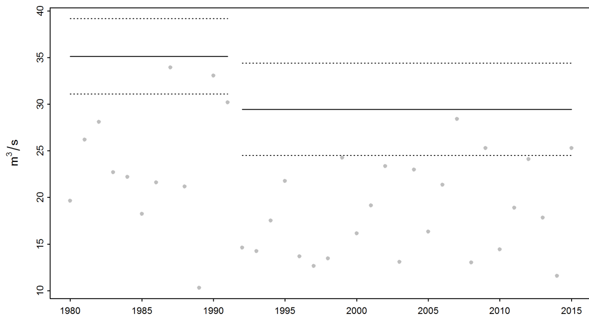
FIGURE 7 – Modification des HQ 100 (calculés à l'aide de la variante «mujump1992») et de l'intervalle de confiance à 95 % (méthode delta ; lignes en traitillé) durant la période 1980-2015
