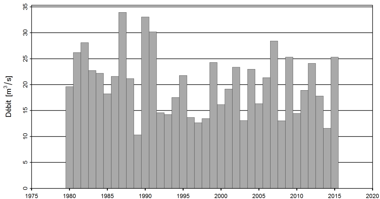
FIGURE 1 – Série chronologique des maxima annuels [ \text{m}^3/\text{s} ] (1980 - 2015, gris foncé : maxima annuels pris en compte)
