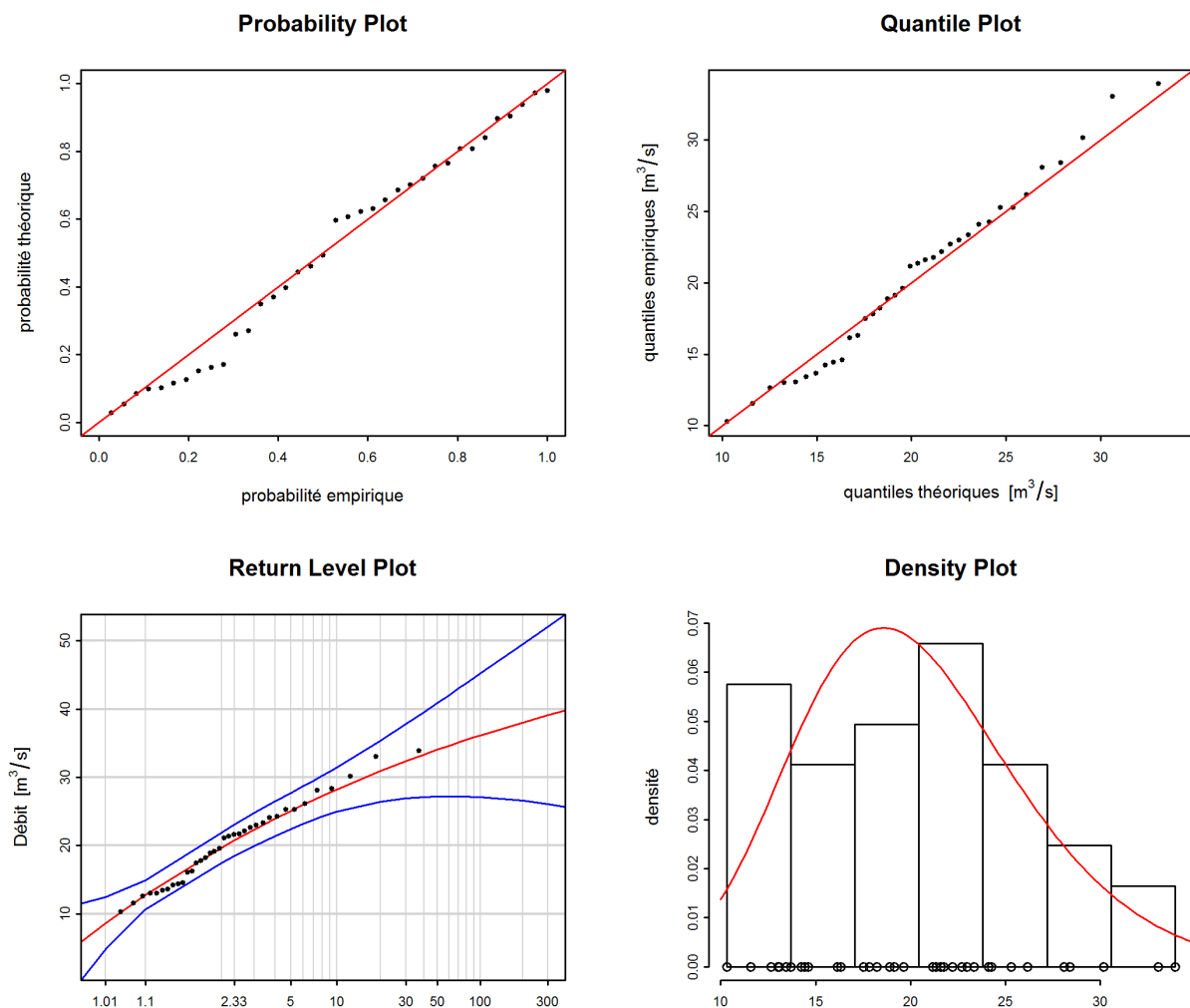
FIGURE 5 – Graphiques diagnostiques de la variante «stat» de la méthode BLOCK(1980-2015)
