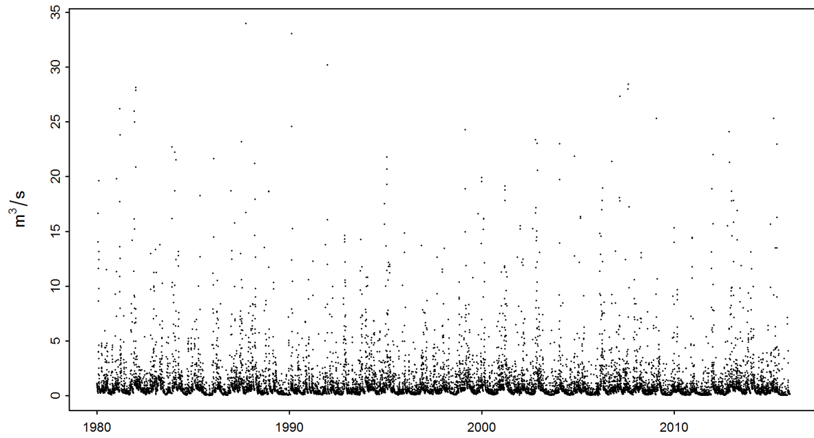
FIGURE 4 – Série chronologique des maxima journaliers [ \text{m}^3/\text{s} ] (01.01.1980 - 31.12.2015)
