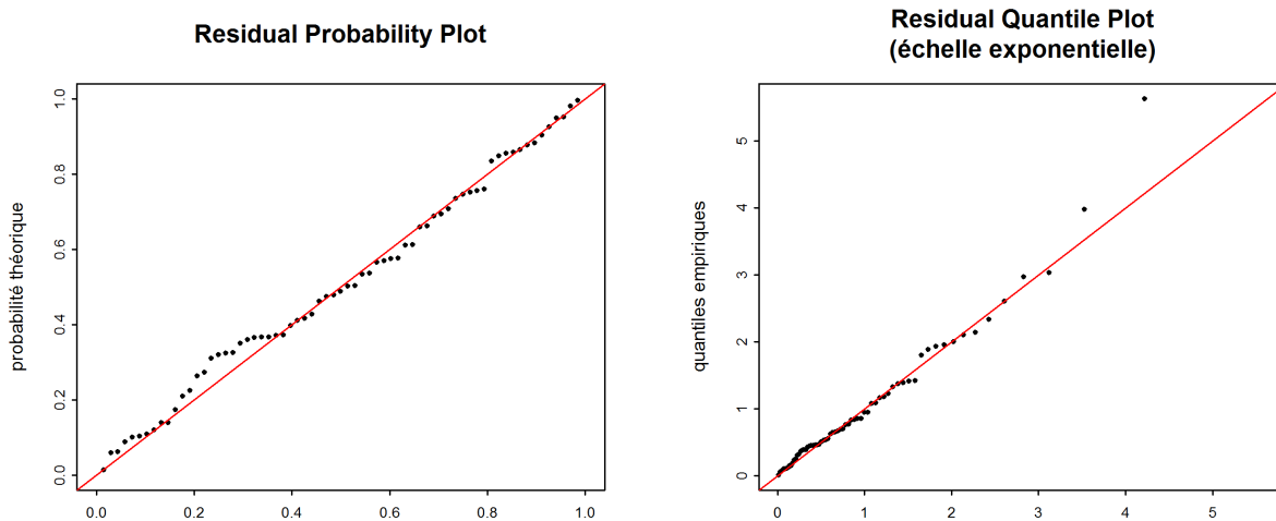
FIGURE 8 – Graphiques diagnostiques de la variante «sigjump2001» de la méthode POT (1979-2015)
