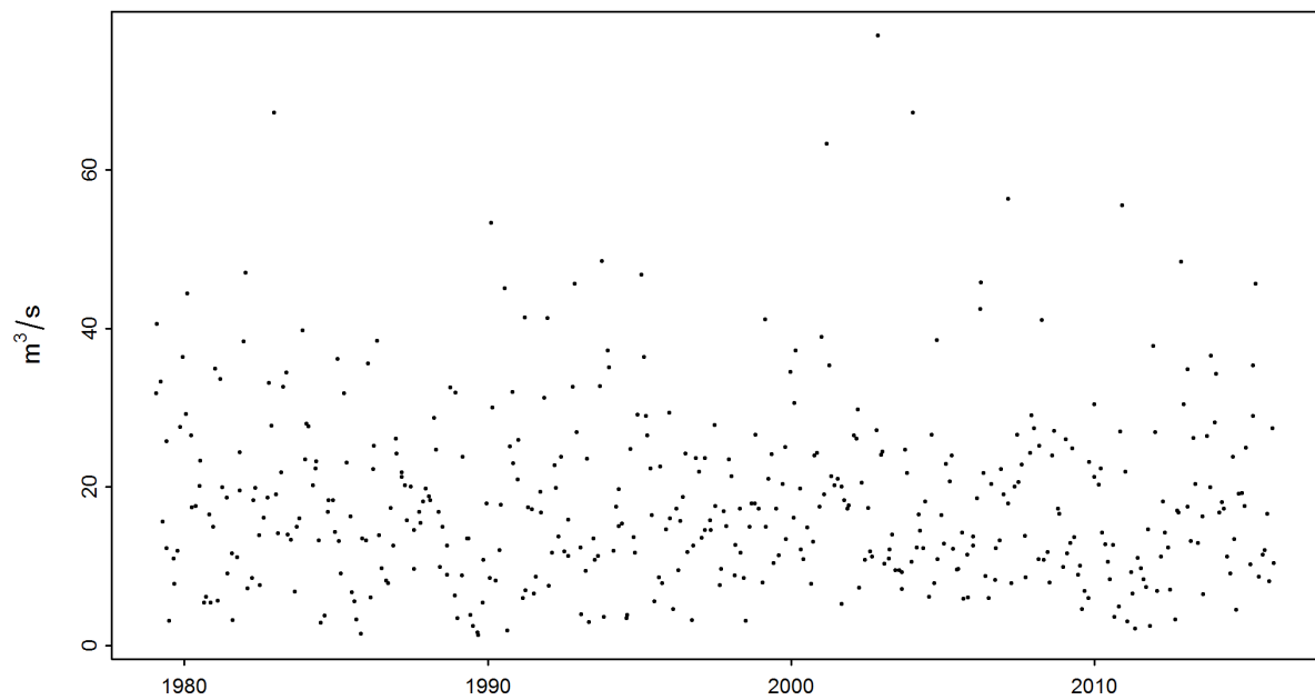
FIGURE 2 – Série chronologique des maxima mensuels [m 3 /s] (01.01.1979 - 31.12.2015)
