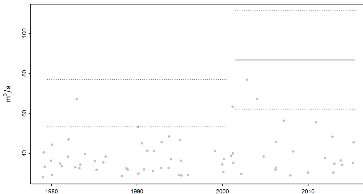
FIGURE 9 – Modification des HQ 100 (calculés à l'aide de la variante «sigjump2001») et de l'intervalle de confiance à 95 % (méthode delta ; lignes en traitillé) durant la période 1979-2015
