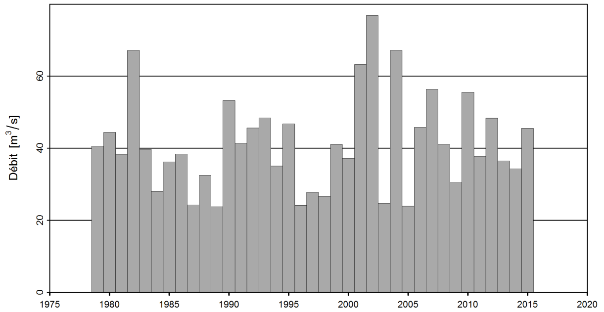
FIGURE 1 – Série chronologique des maxima annuels [m 3 /s] (1979 - 2015, gris foncé : maxima annuels pris en compte)
