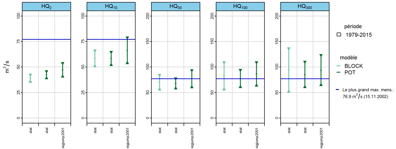
FIGURE 10 – HQ_T [ m^3/s ] y c. un intervalle de confiance à 95 % calculé à l'aide du modèle stationnaire ainsi qu'au moyen de la meilleure variante de la méthode BLOCK et POT pour l'année 2015
