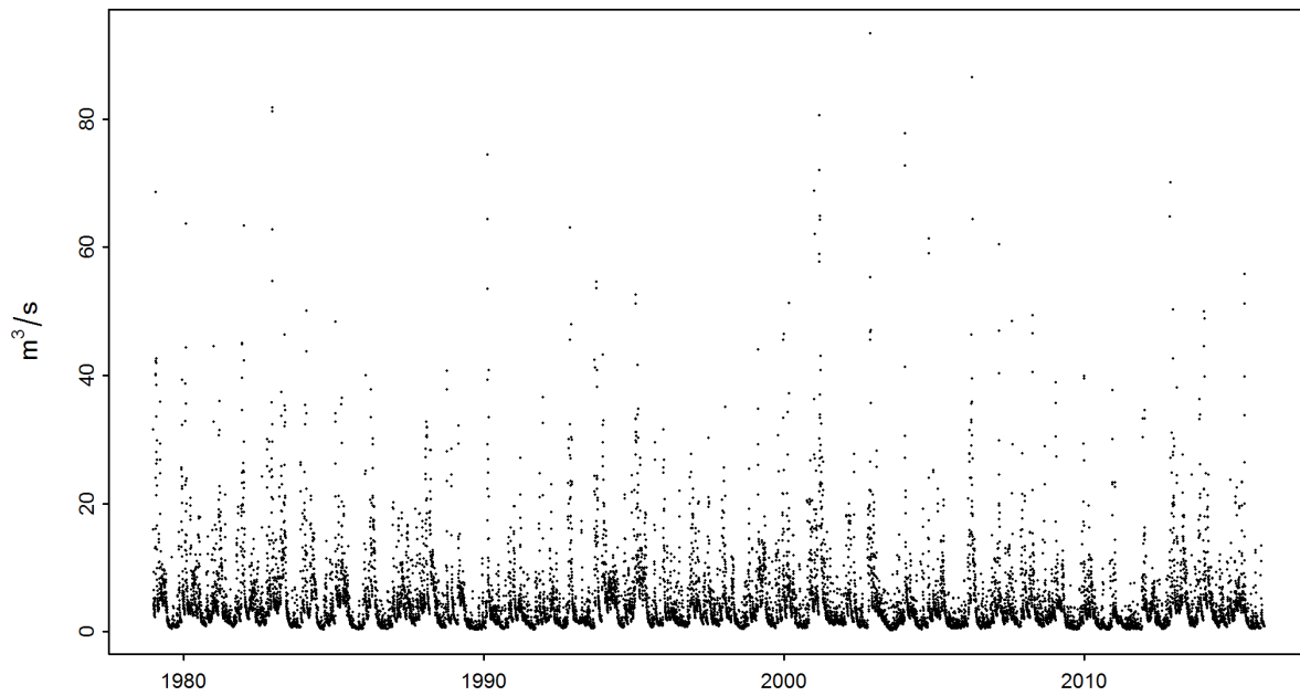
FIGURE 4 – Série chronologique des maxima journaliers [m 3 /s] (01.01.1979 - 31.12.2015)
