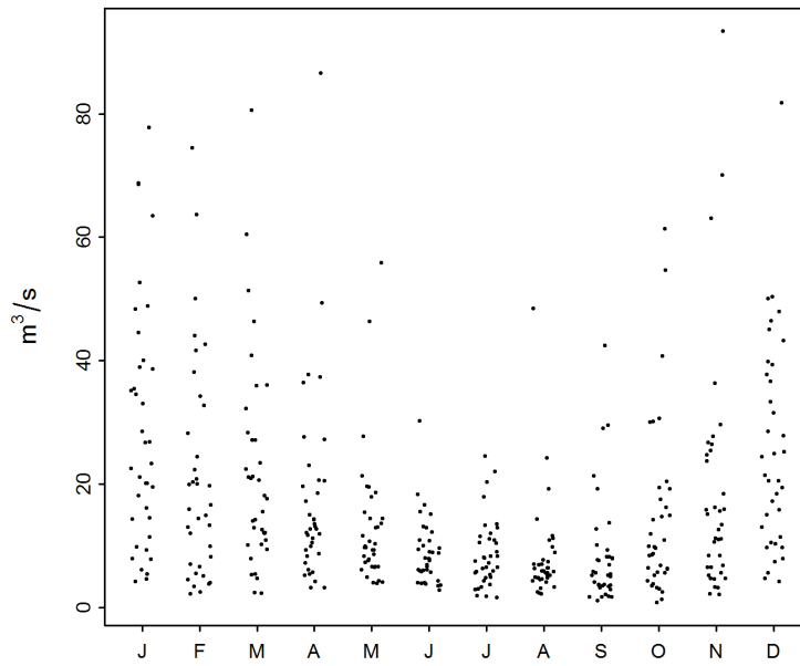
FIGURE 3 – Variations saisonnières des maxima mensuels [m 3 /s] (01.01.1979 - 31.12.2015)
