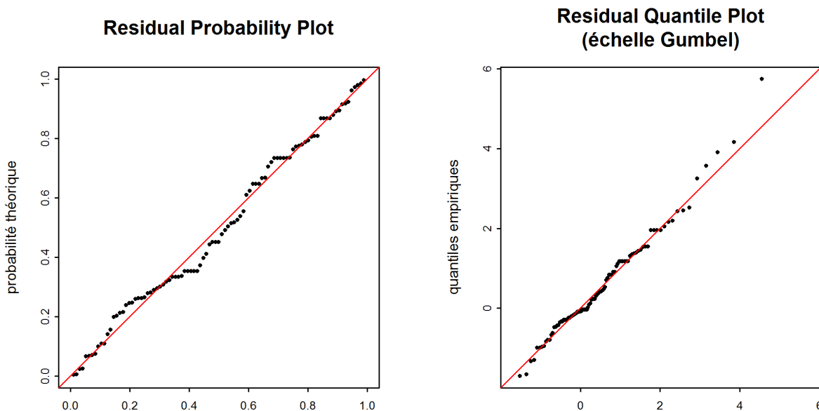
FIGURE 6 – Graphiques diagnostiques de la variante «mujump1971» de la méthode BLOCK (1921-2015)
