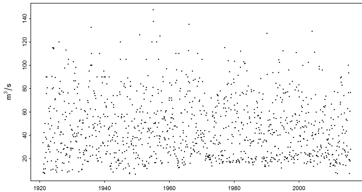
FIGURE 2 – Série chronologique des maxima mensuels [m 3 /s] (01.01.1921 - 31.12.2015)
