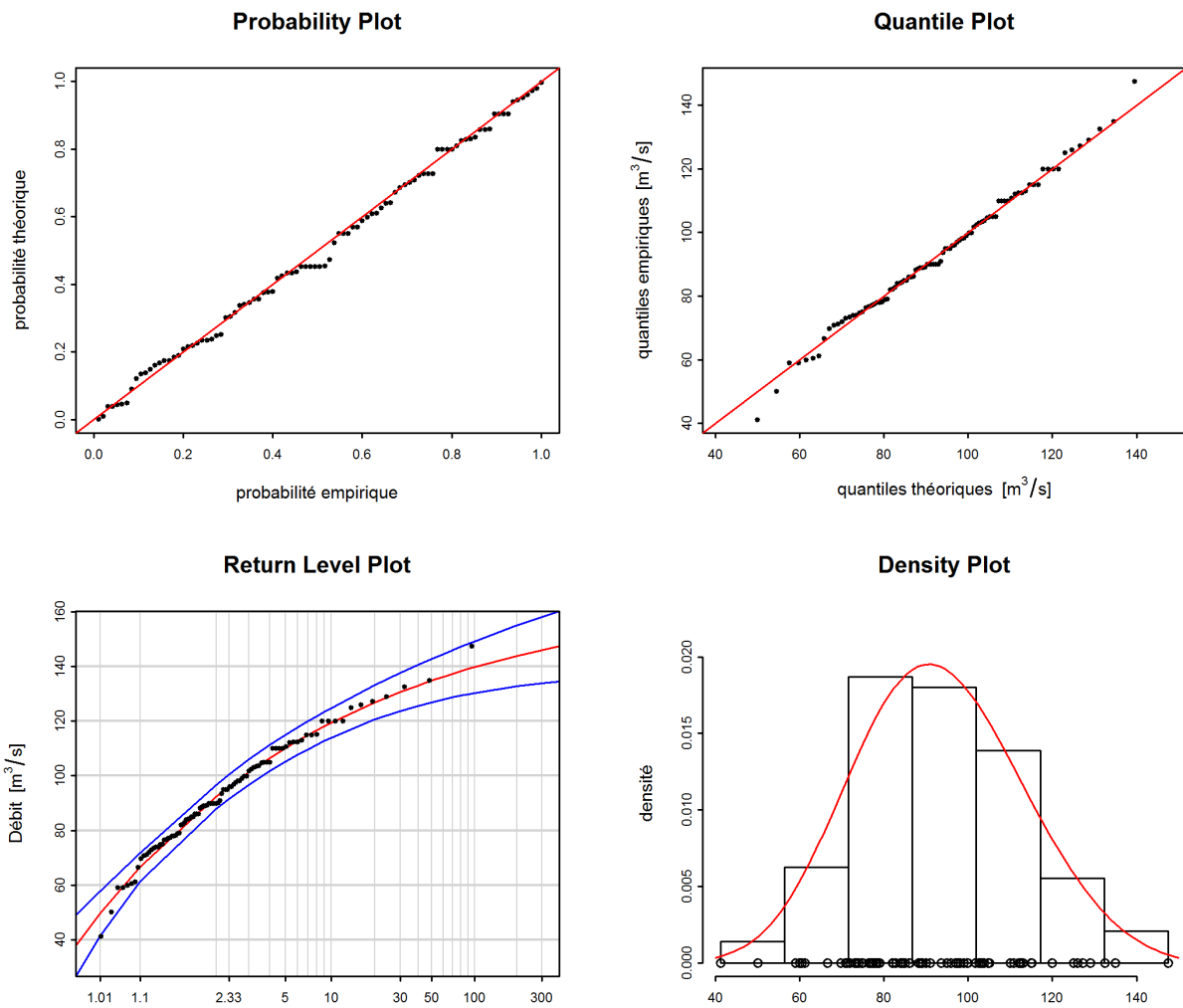
FIGURE 5 – Graphiques diagnostiques de la variante «stat» de la méthode BLOCK(1921-2015)
