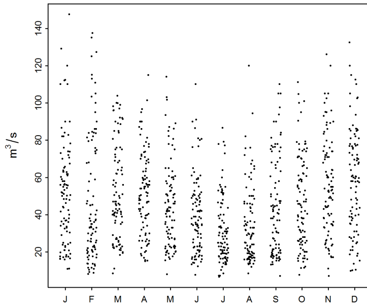
FIGURE 3 – Variations saisonnières des maxima mensuels [ \text{m}^3/\text{s} ] (01.01.1921 - 31.12.2015)
