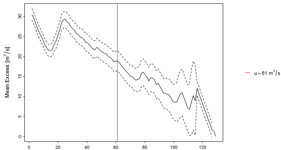
FIGURE 12 – «mean residual life plot» avec le seuil déterminé u (ligne rouge), dépassement moyen (ligne noire), intervalle de confiance à 95 % (traitillés)
