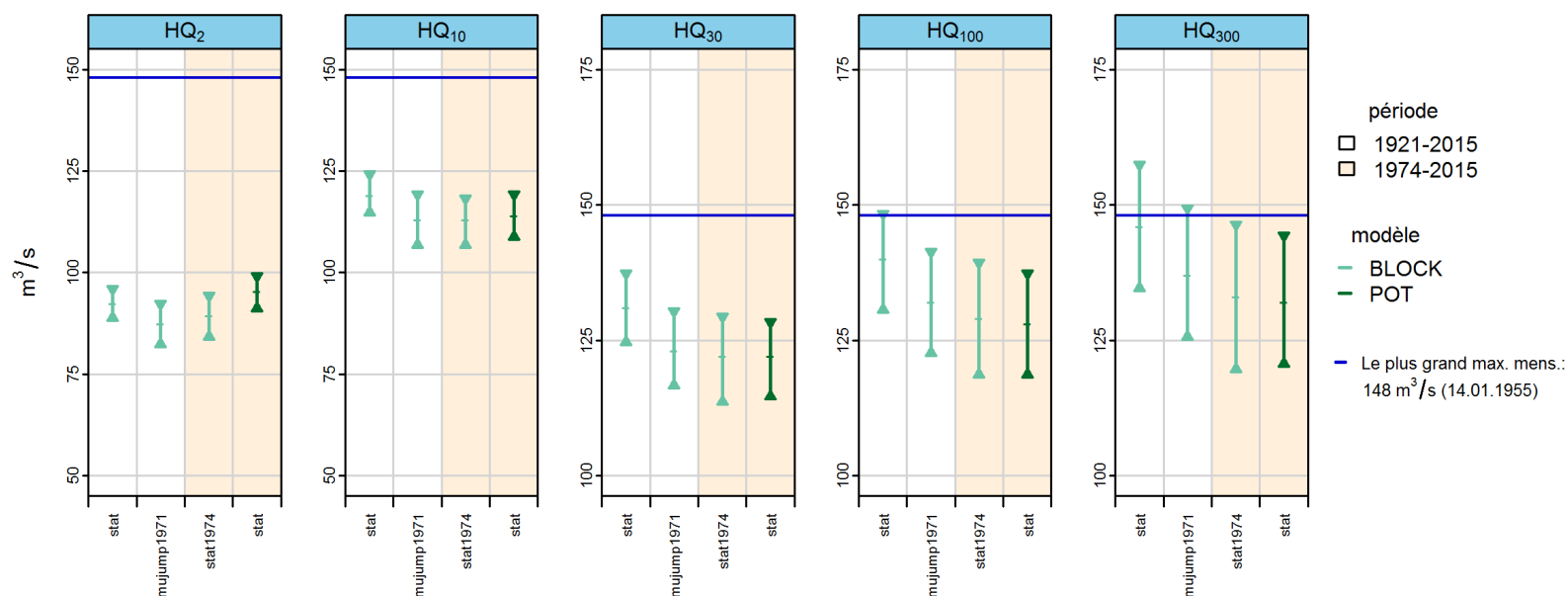
FIGURE 11 – HQ T [m 3 /s] y c. un intervalle de confiance à 95 % calculé à l'aide du modèle stationnaire ainsi qu'au moyen de la meilleure variante de la méthode BLOCK et POT pour l'année 2015
