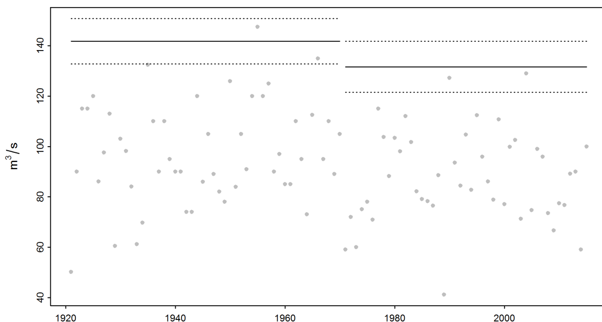
FIGURE 7 – Modification des HQ 100 (calculés à l'aide de la variante «mujump1971») et de l'intervalle de confiance à 95 % (méthode delta ; lignes en traitillé) durant la période 1921-2015
