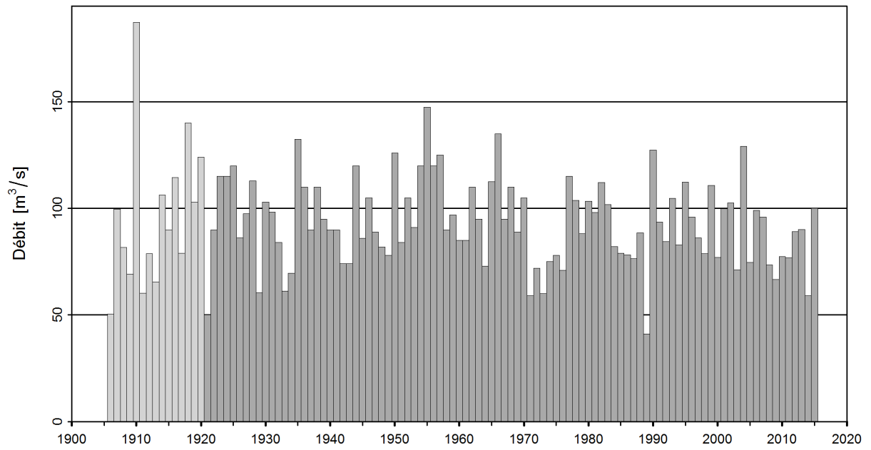
FIGURE 1 – Série chronologique des maxima annuels [m 3 /s] (1906 - 2015, Gris clair : maxima non pris en compte dans la statistique, gris foncé : maxima annuels pris en compte)
