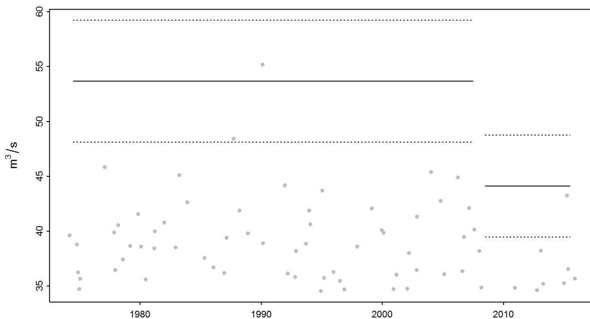
FIGURE 12 – Modification des HQ 100 (calculés à l'aide de la variante «sigjump2008») et de l'intervalle de confiance à 95 % (méthode delta ; lignes en traitillé) durant la période 1974-2015
