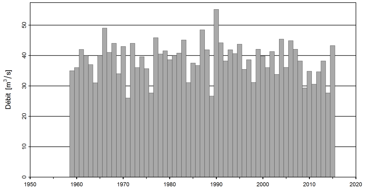
FIGURE 1 – Série chronologique des maxima annuels [ \text{m}^3/\text{s} ] (1959 - 2015, gris foncé : maxima annuels pris en compte)
