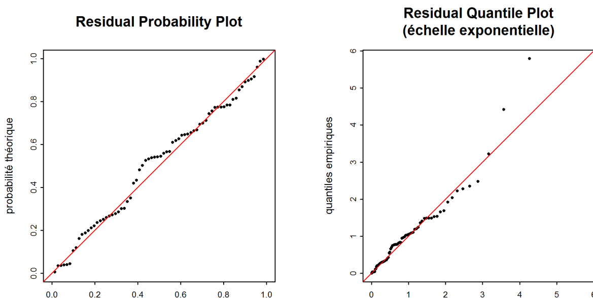
FIGURE 11 – Graphiques diagnostiques de la variante «sigjump2008» de la méthode POT (1974-2015)
