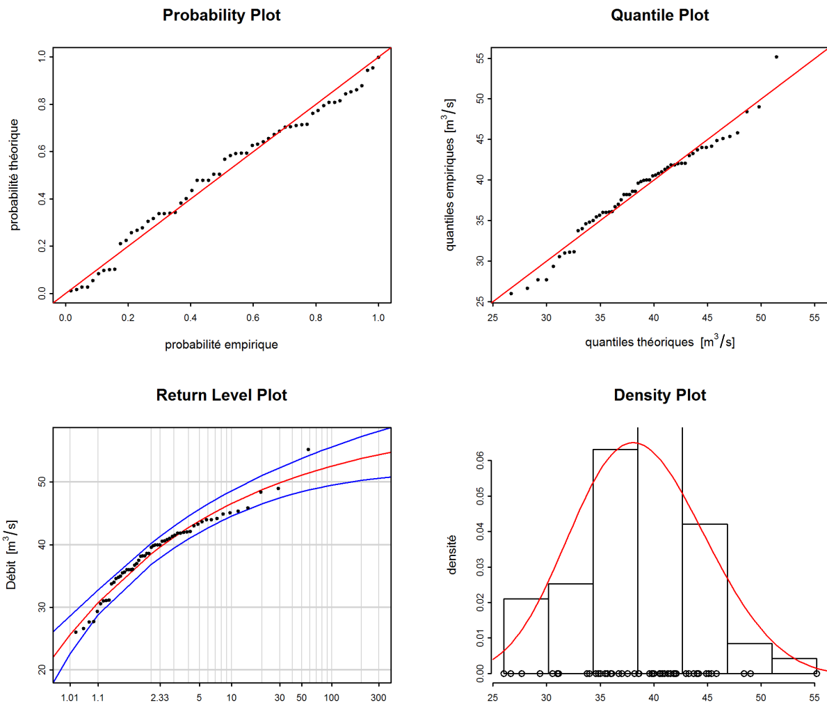
FIGURE 5 – Graphiques diagnostiques de la variante «stat» de la méthode BLOCK(1959-2015)
