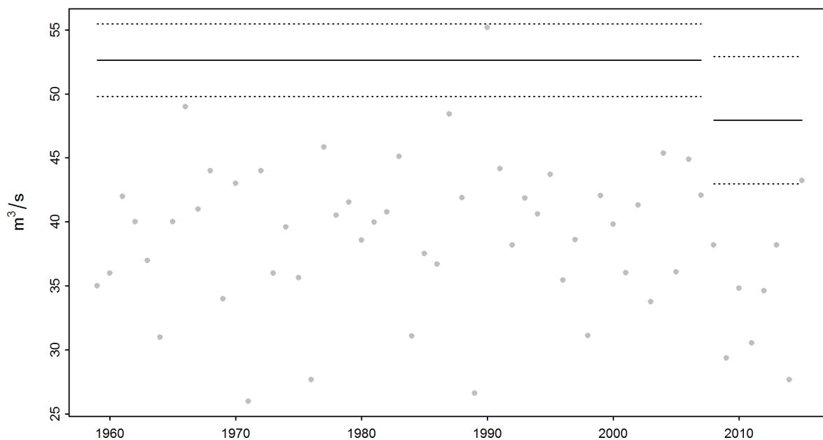
FIGURE 7 – Modification des HQ 100 (calculés à l'aide de la variante «mujump2008») et de l'intervalle de confiance à 95 % (méthode delta ; lignes en traitillé) durant la période 1959-2015
