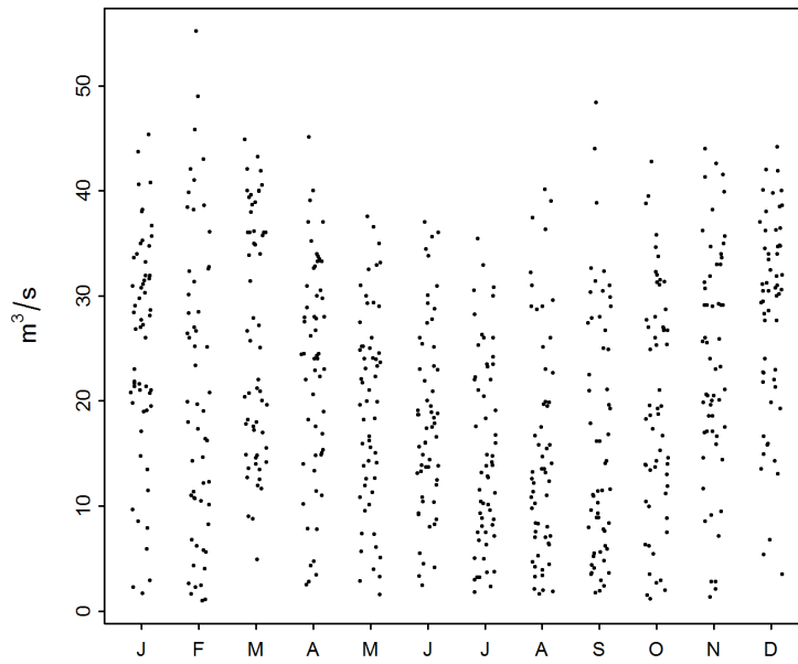
FIGURE 3 – Variations saisonnières des maxima mensuels [ \text{m}^3/\text{s} ] (01.01.1959 - 31.12.2015)
