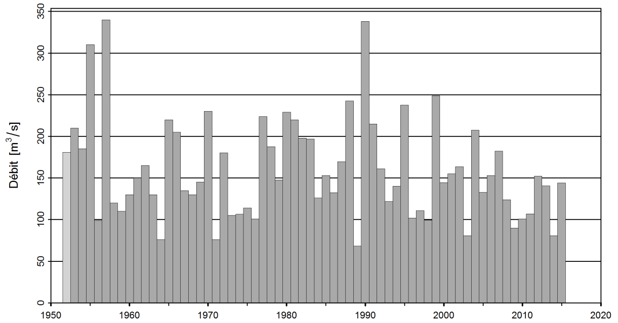
FIGURE 1 – Série chronologique des maxima annuels [ \text{m}^3/\text{s} ] (1952 - 2015, Gris clair : maxima non pris en compte dans la statistique, gris foncé : maxima annuels pris en compte)
