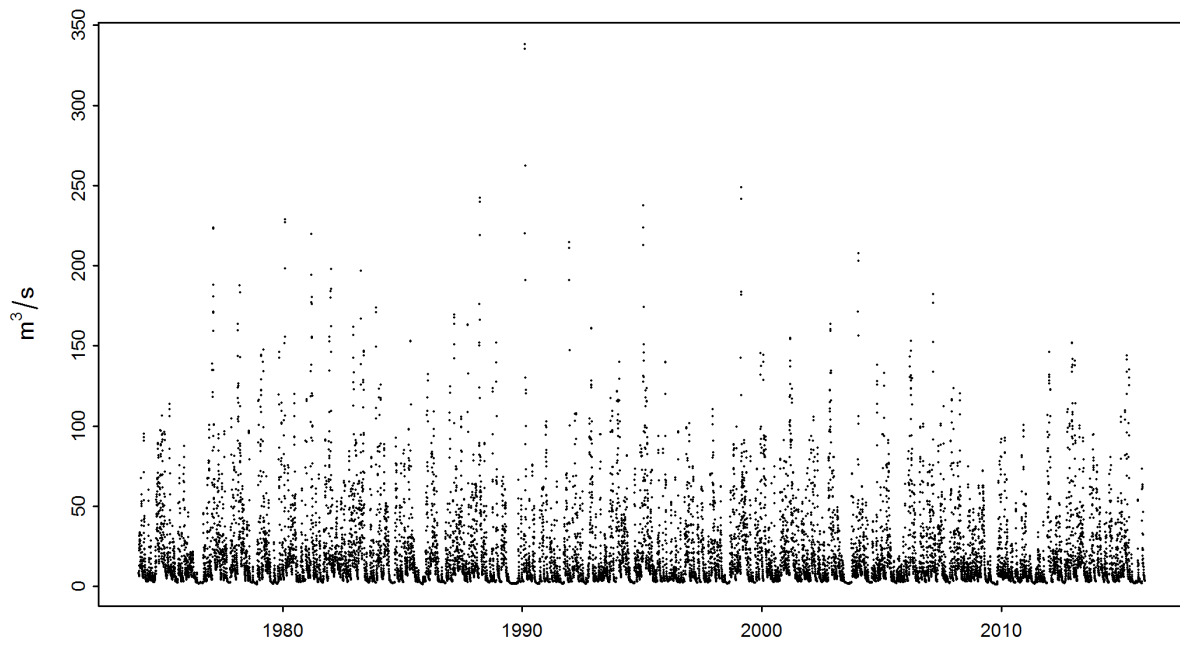
FIGURE 4 – Série chronologique des maxima journaliers [m 3 /s] (01.01.1974 - 31.12.2015)
