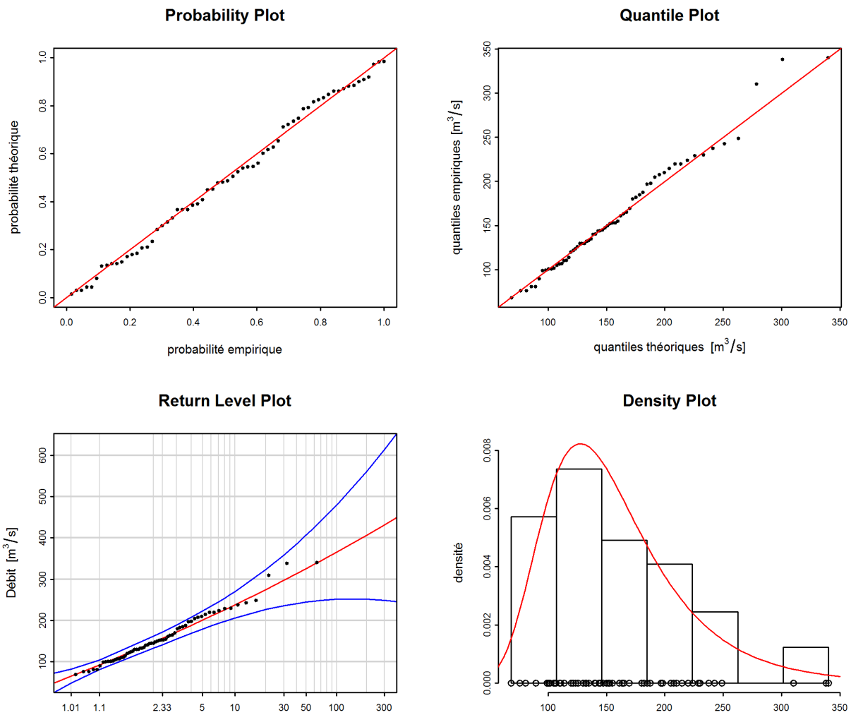
FIGURE 5 – Graphiques diagnostiques de la variante «stat» de la méthode BLOCK(1953-2015)
