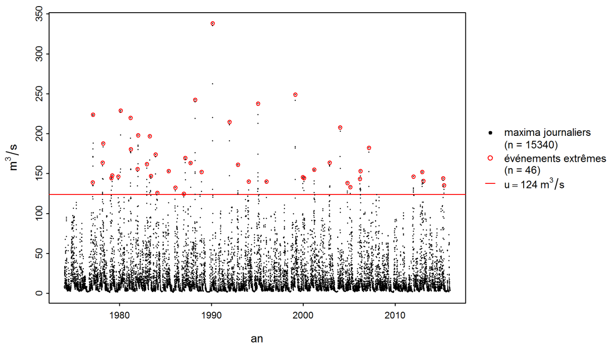
FIGURE 7 – Sélection des valeurs extrêmes utilisées dans la méthode POT
