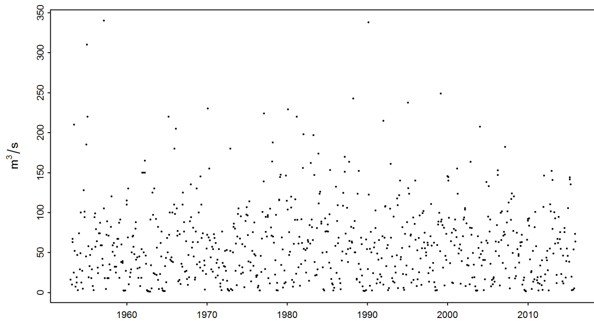
FIGURE 2 – Série chronologique des maxima mensuels [ \text{m}^3/\text{s} ] (01.01.1953 - 31.12.2015)
