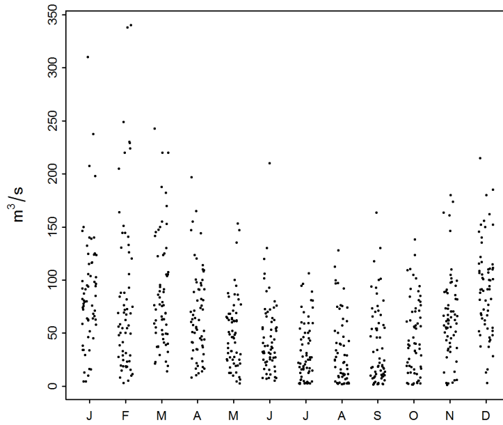
FIGURE 3 – Variations saisonnières des maxima mensuels [m 3 /s] (01.01.1953 - 31.12.2015)
