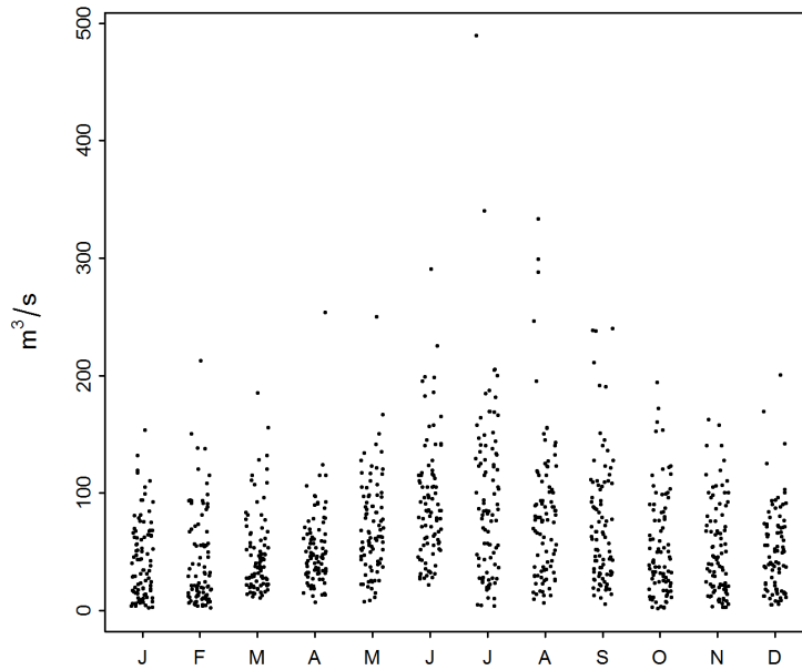
Abbildung 3: Saisonaler Verlauf der Monatsmaxima [ \text{m}^3/\text{s} ] (01.01.1928 - 31.12.2015)
