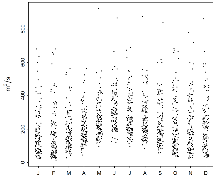
FIGURE 3 – Variations saisonnières des maxima mensuels [ \text{m}^3/\text{s} ] (01.01.1904 - 31.12.2015)
