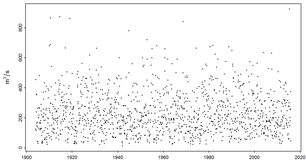
FIGURE 2 – Série chronologique des maxima mensuels [ \text{m}^3/\text{s} ] (01.01.1904 - 31.12.2015)
