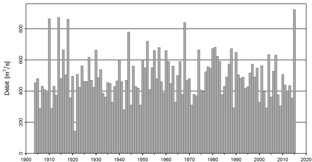
FIGURE 1 – Série chronologique des maxima annuels [ \text{m}^3/\text{s} ] (1904 - 2015, gris foncé : maxima annuels pris en compte)
