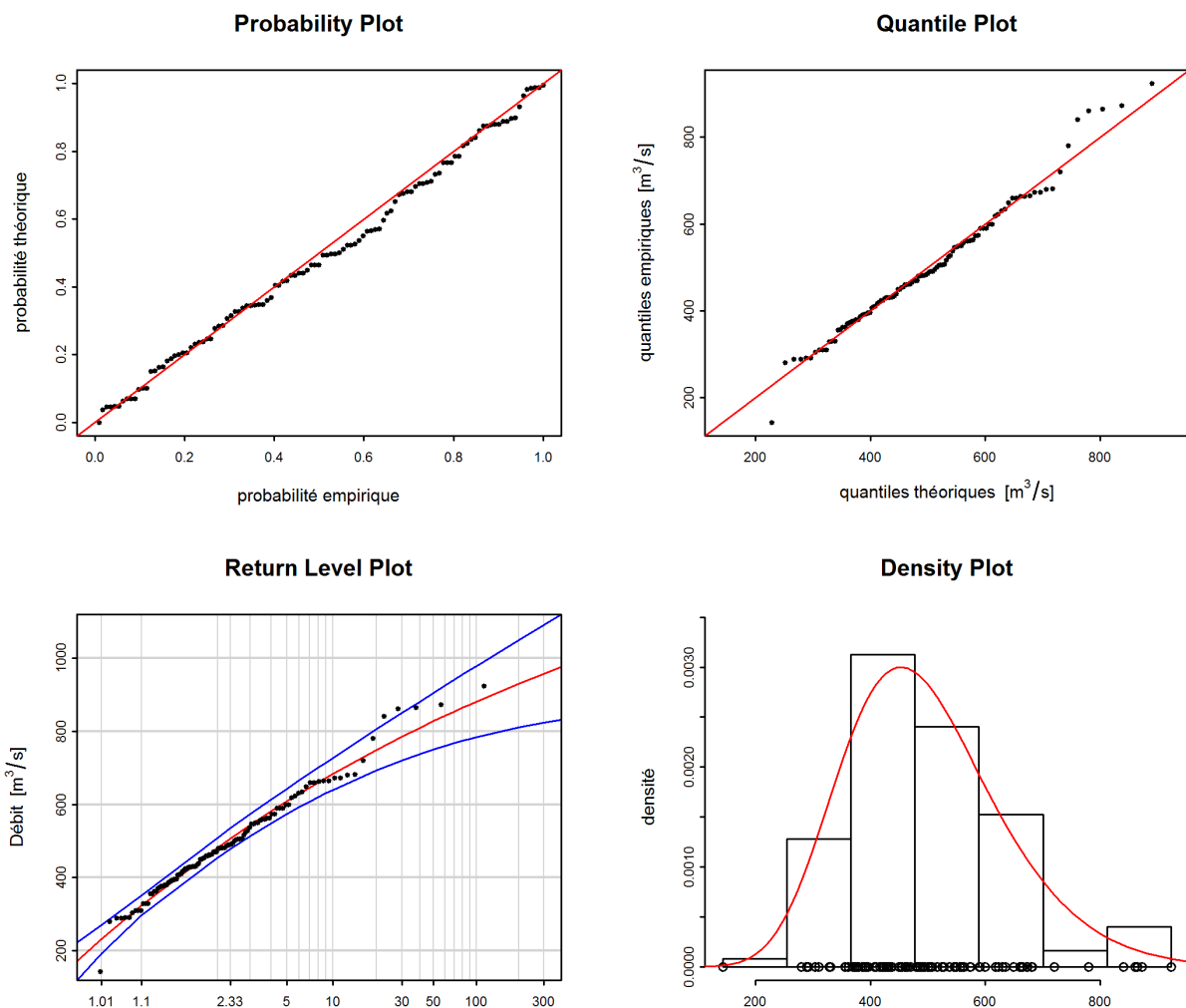
FIGURE 5 – Graphiques diagnostiques de la variante «stat» de la méthode BLOCK(1904-2015)
