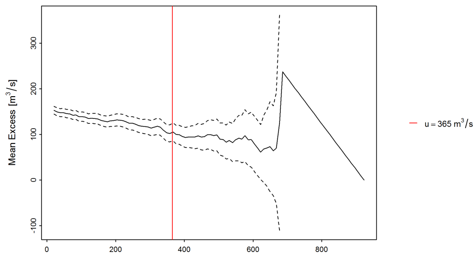
FIGURE 10 – «mean residual life plot» avec le seuil déterminé u (ligne rouge), dépassement moyen (ligne noire), intervalle de confiance à 95 % (traitillés)
