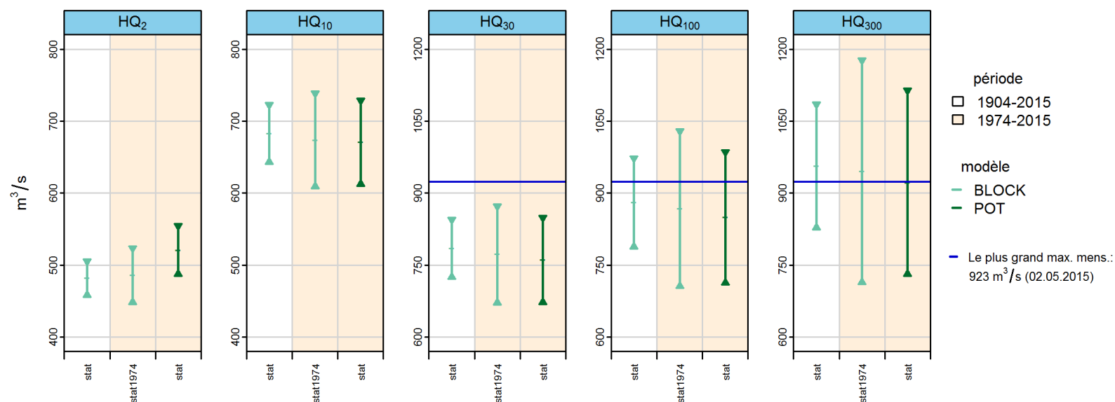
FIGURE 9 – HQ T [m³/s] y c. un intervalle de confiance à 95 % calculé à l'aide du modèle stationnaire ainsi qu'au moyen de la meilleure variante de la méthode BLOCK et POT pour l'année 2015
