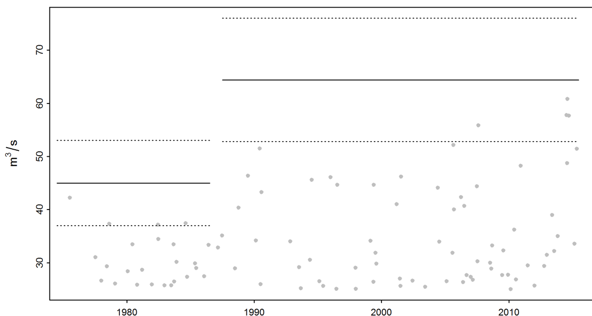
Abbildung 12: Veränderung der mit der Modellvariante „sigjump1987“ berechneten HQ 100 (durchgezogene Linien) und des 95%-Konfidenzintervalls (Deltamethode; gestrichelte Linien) über die Jahre 1974-2015
