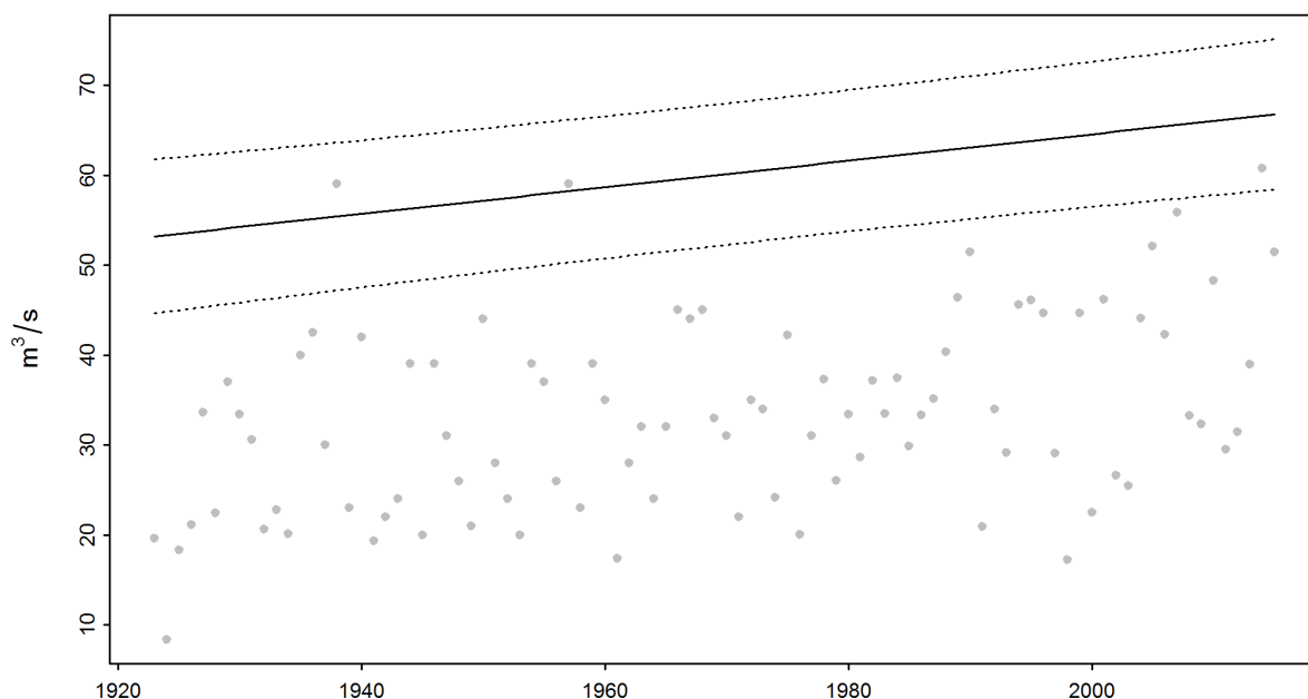
Abbildung 7: Veränderung der mit der Modellvariante „mul“ berechneten HQ 100 (durchgezogene Linien) und des 95%-Konfidenzintervalls (Deltamethode; gestrichelte Linien) über die Jahre 1923-2015
