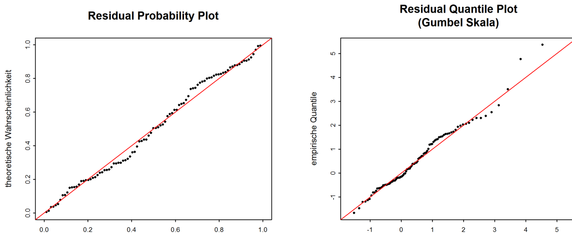
Abbildung 6: Diagnostikplots der Modellvariante „mul“ des BLOCK-Ansatzes (1923-2015)
