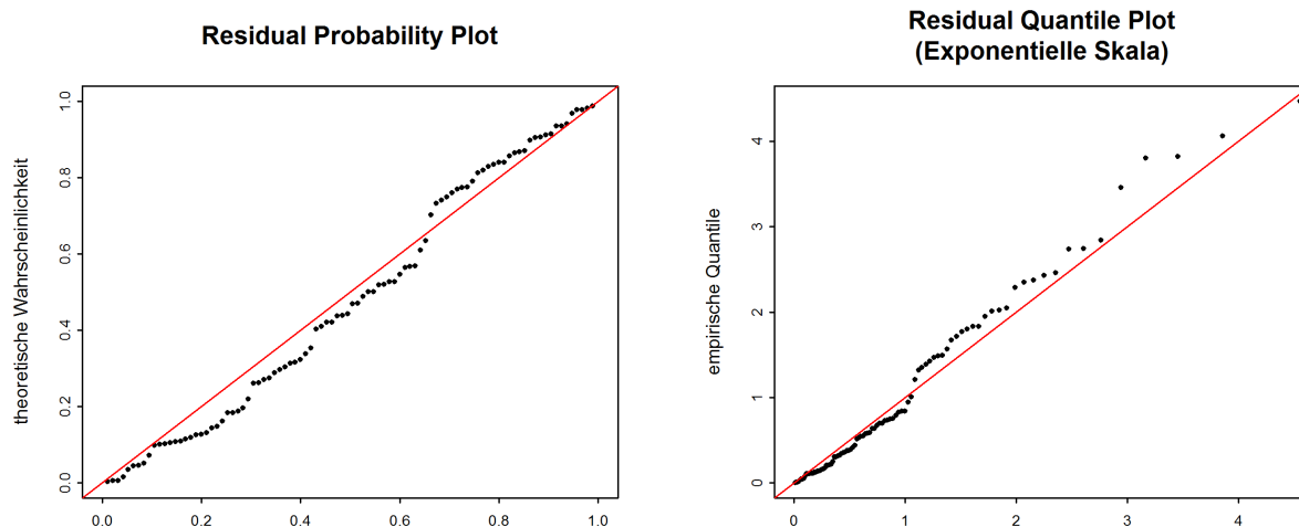
Abbildung 11: Diagnostikplots der Modellvariante „sigjump1987“ des POT-Ansatzes (1974-2015)
