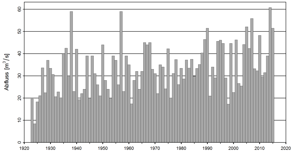
Abbildung 1: Zeitreihe der Jahresmaxima [m 3 /s] (1922 - 2015, dunkelgrau: verwendete Jahresmaxima)
