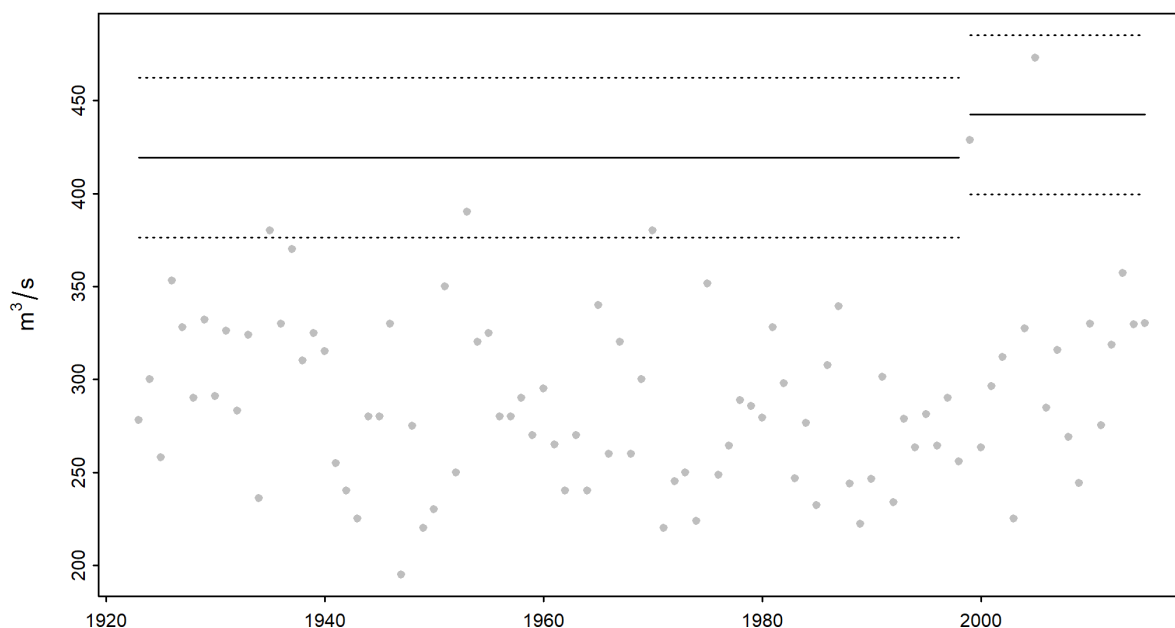
Abbildung 7: Veränderung der mit der Modellvariante „mujump1999“ berechneten HQ 100 (durchgezogene Linien) und des 95%-Konfidenzintervalls (Deltamethode; gestrichelte Linien) über die Jahre 1923-2015
