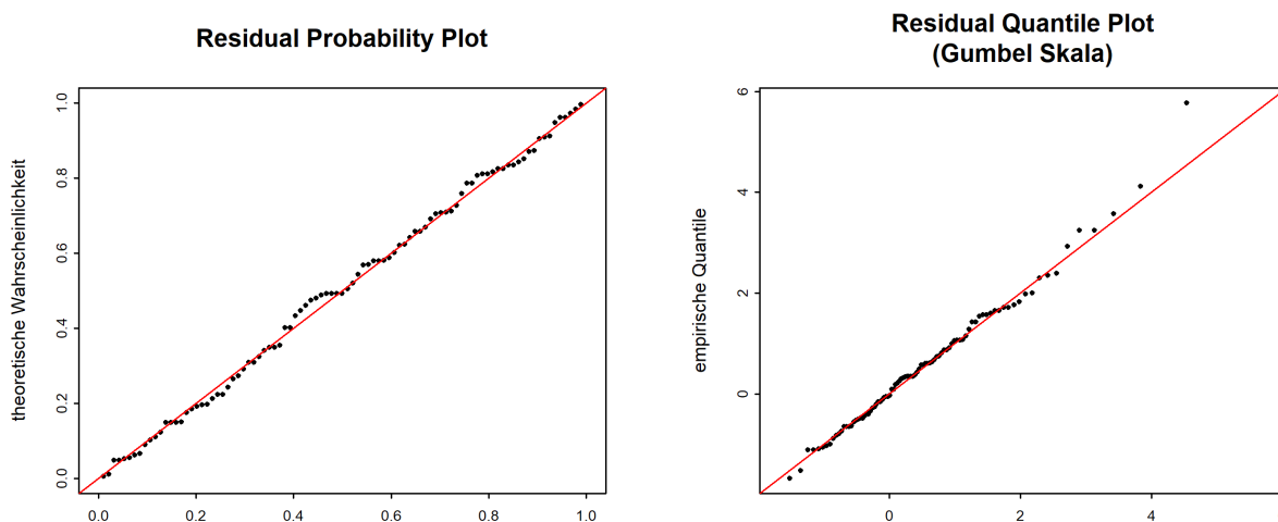
Abbildung 6: Diagnostikplots der Modellvariante „mujump1999“ des BLOCK-Ansatzes (1923-2015)
