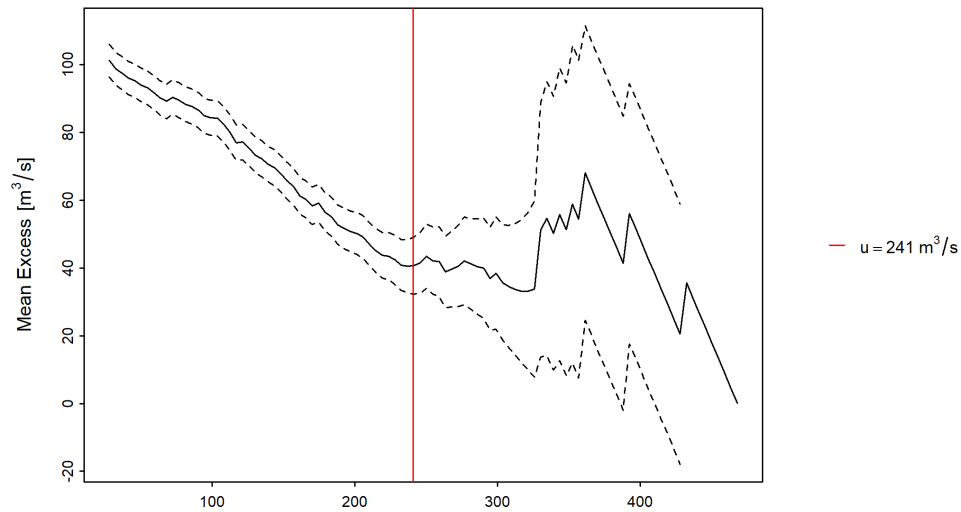
Abbildung 12: „mean residual life plot“ mit gewählttem Schwellenwert u (rote Linie) mean Excess (schwarze Linie), 95%-Konfidenzintervall (gestrichelte Linien)
