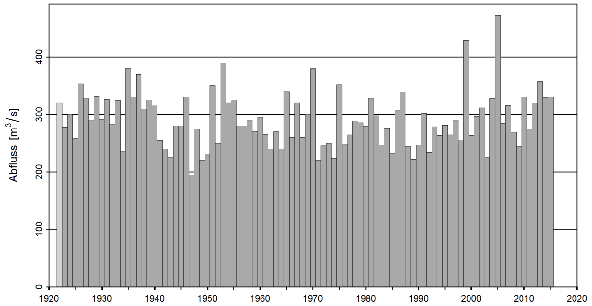
Abbildung 1: Zeitreihe der Jahresmaxima [ \text{m}^3/\text{s} ] (1922 - 2015, hellgrau: nicht für die Statistik verwendetes Jahresmaximum, dunkelgrau: verwendete Jahresmaxima der gesamten Auswertungsperiode ab Limnigrapheninstallation).
