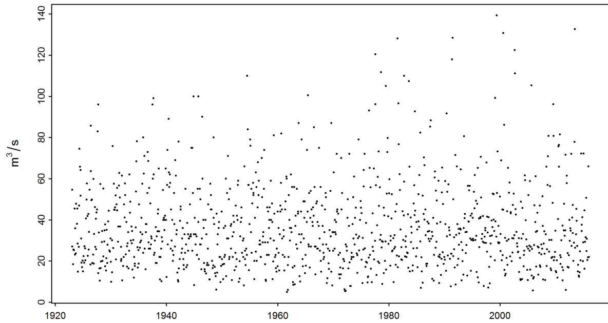
Abbildung 2: Zeitreihe der Monatsmaxima [m 3 /s] (01.01.1923 - 31.12.2015)
