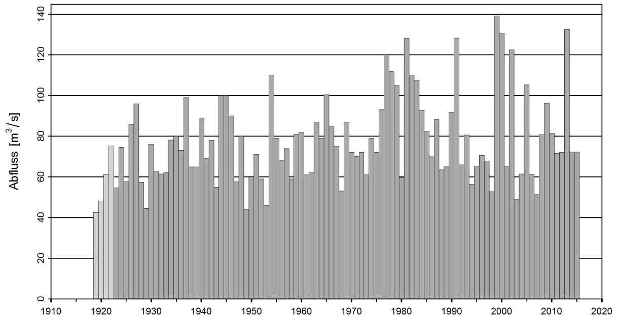
Abbildung 1: Zeitreihe der Jahresmaxima [m 3 /s] (1919 - 2015, hellgrau: nicht für die Statistik verwendete Jahresmaxima, dunkelgrau: verwendete Jahresmaxima)
