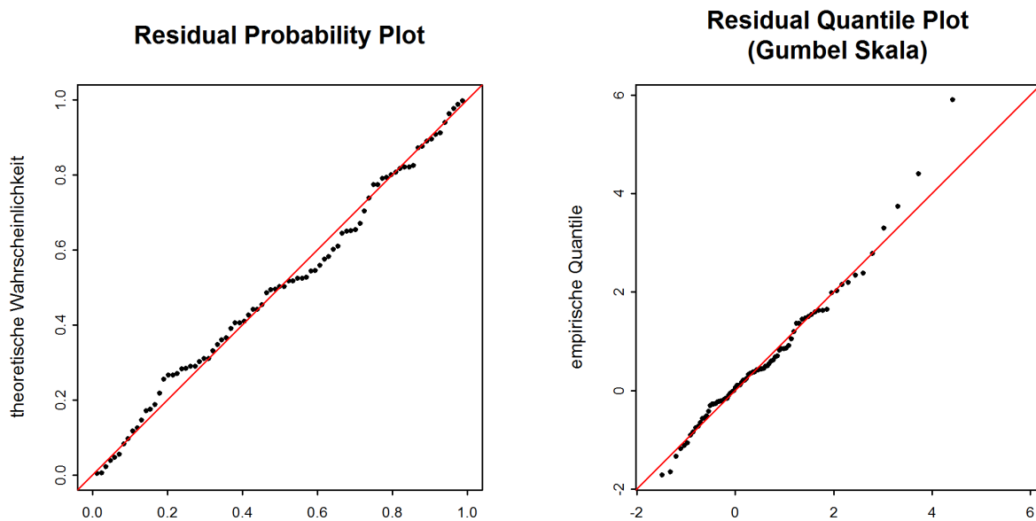
Abbildung 6: Diagnostikplots der Modellvariante „mujump1968“ des BLOCK-Ansatzes (1933-2015)
