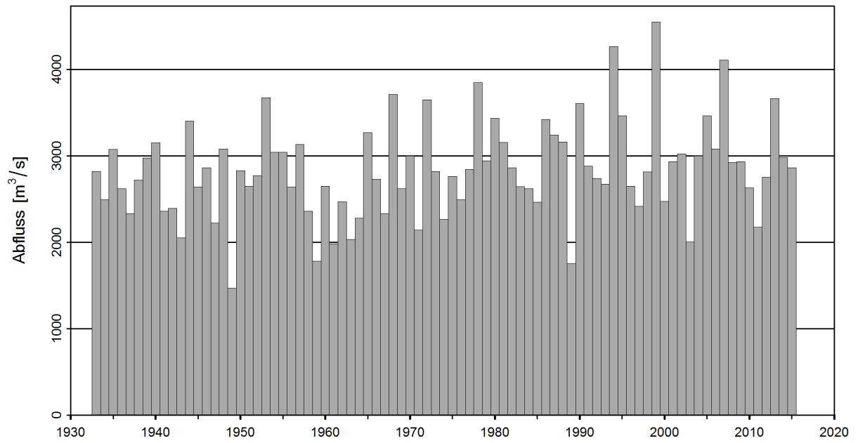
Abbildung 1: Zeitreihe der Jahresmaxima [m³/s] (1933 - 2015, dunkelgrau: verwendete Jahresmaxima)
