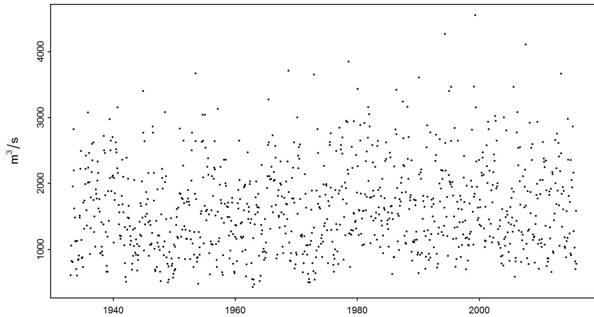
Abbildung 2: Zeitreihe der Monatsmaxima [m³/s] (01.01.1933 - 31.12.2015)
