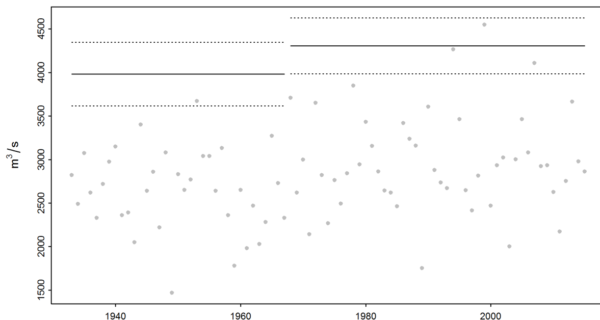
Abbildung 7: Veränderung der mit der Modellvariante „mujump1968“ berechneten HQ 100 (durchgezogene Linien) und des 95%-Konfidenzintervalls (Deltamethode; gestrichelte Linien) über die Jahre 1933-2015
