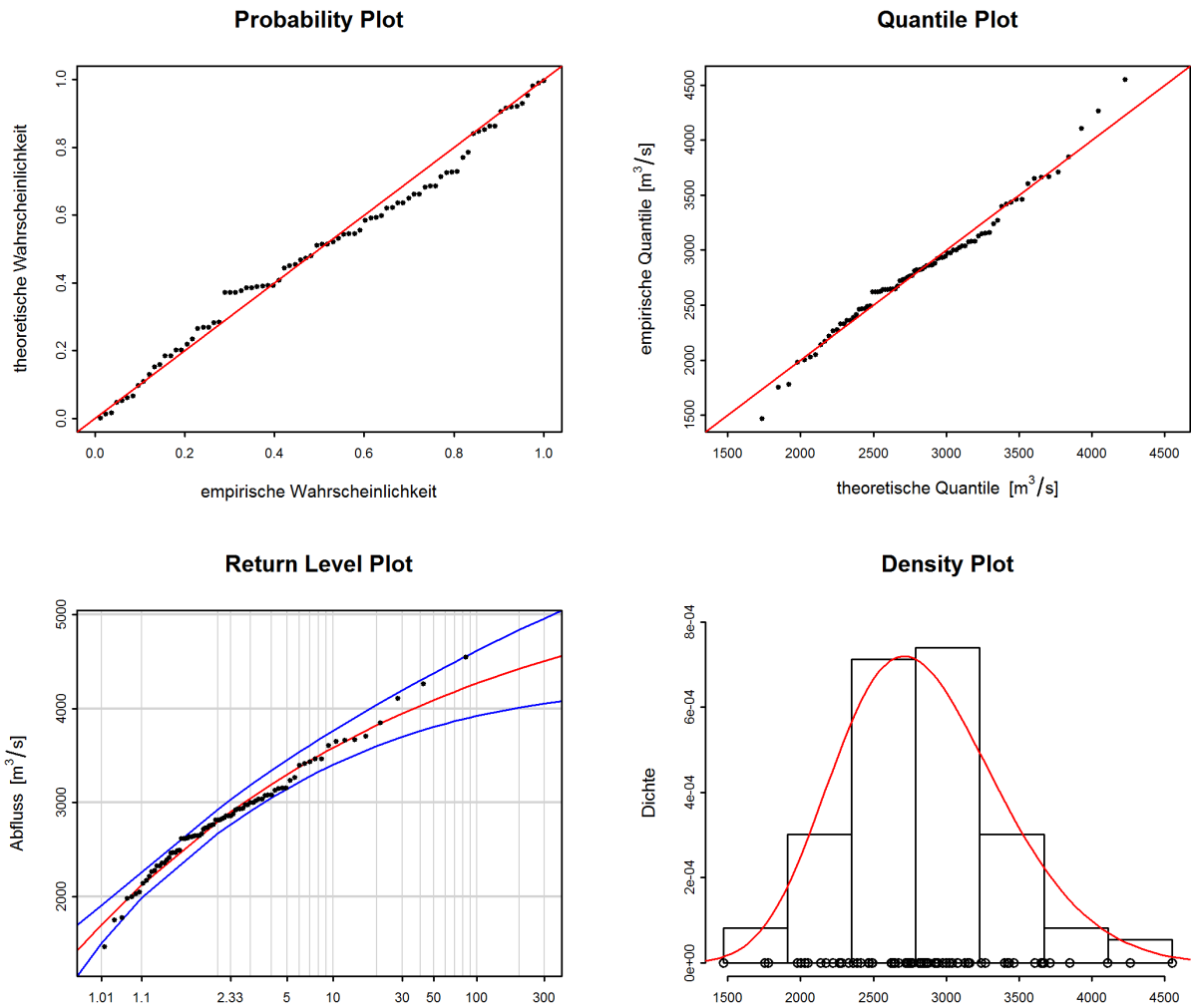
Abbildung 5: Diagnostikplots der Modellvariante „stat“ des BLOCK-Ansatzes (1933-2015)
