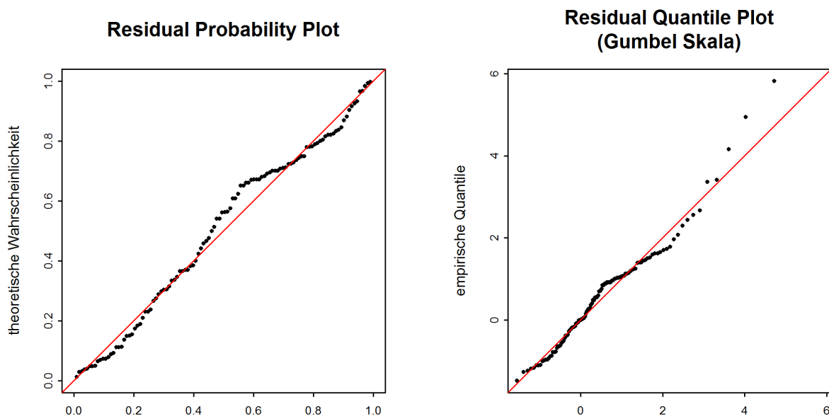
Abbildung 6: Diagnostikplots der Modellvariante „mujump1964“ des BLOCK-Ansatzes (1904-2015)
