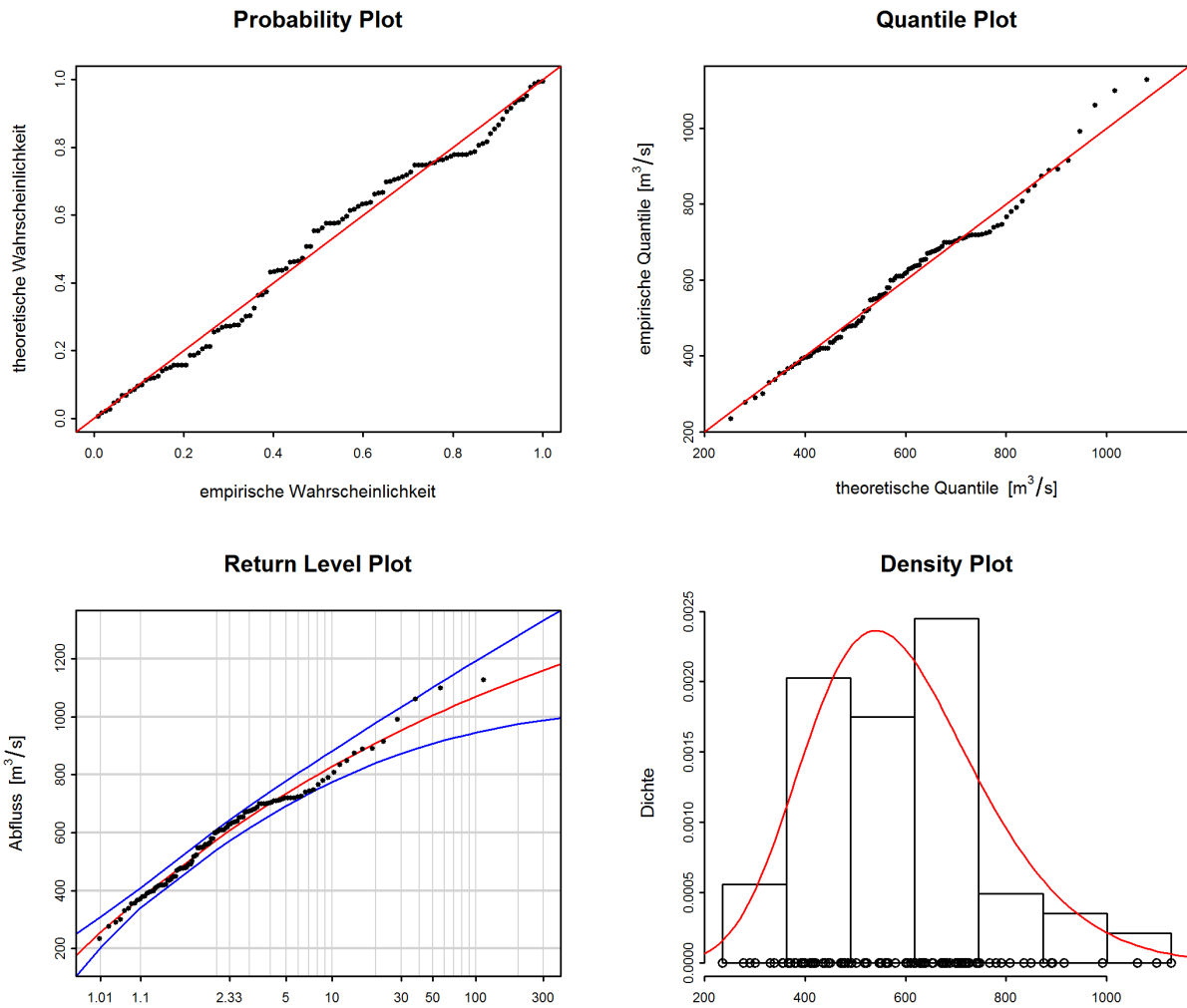
Abbildung 5: Diagnostikplots der Modellvariante „stat“ des BLOCK-Ansatzes (1904-2015)
