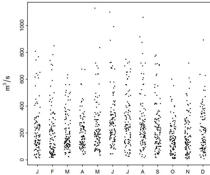
Abbildung 3: Saisonaler Verlauf der Monatsmaxima [ \text{m}^3/\text{s} ] (01.01.1904 - 31.12.2015)
