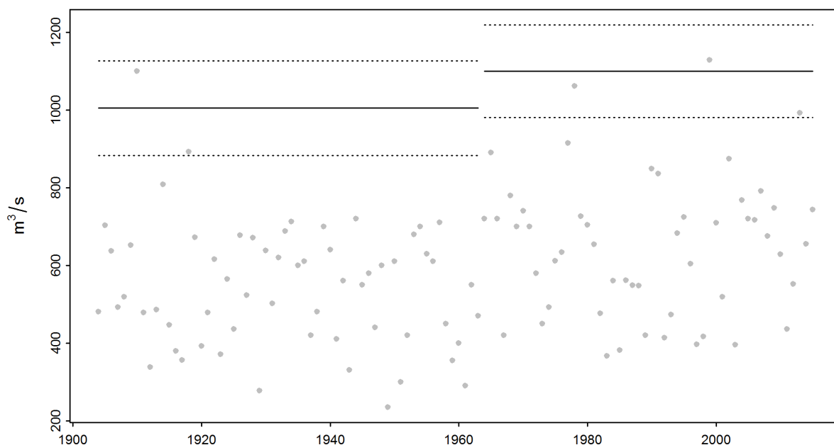
Abbildung 7: Veränderung der mit der Modellvariante „mujump1964“ berechneten HQ 100 (durchgezogene Linien) und des 95%-Konfidenzintervalls (Deltamethode; gestrichelte Linien) über die Jahre 1904-2015
