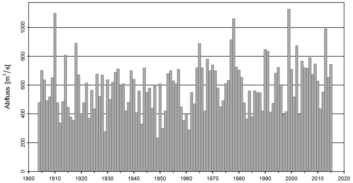
Abbildung 1: Zeitreihe der Jahresmaxima [m 3 /s] (1904 - 2015, dunkelgrau: verwendete Jahresmaxima)
