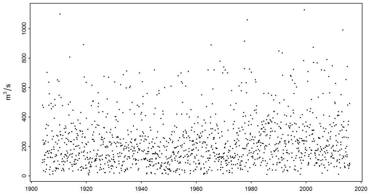
Abbildung 2: Zeitreihe der Monatsmaxima [m 3 /s] (01.01.1904 - 31.12.2015)
