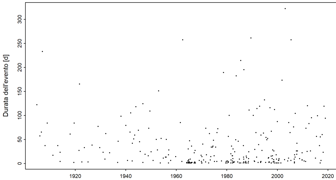
Figura 4: Serie temporale della durata di magra [d] (01.06.1901 - 31.05.2019)
