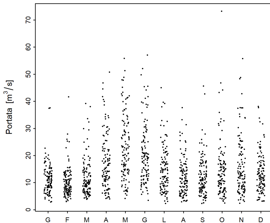
Figura 2: Sviluppo stagionale del minimo mensile di M7Q [ \text{m}^3/\text{s} ] (01.06.1901 - 31.05.2019)
