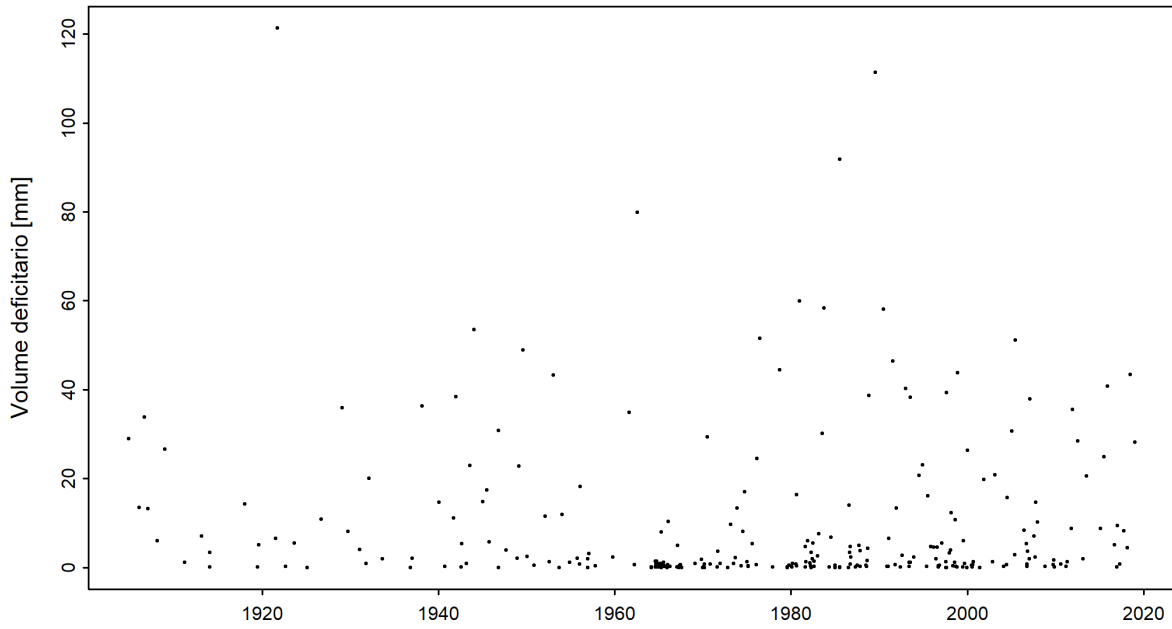
Figura 5: Serie temporale del volume deficitario [mm] (01.06.1901 - 31.05.2019)
