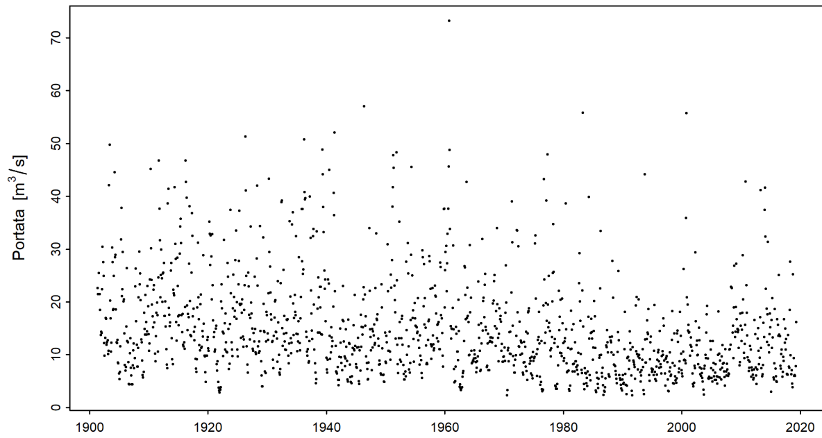
Figura 3: Serie temporale del minimo mensile di M7Q [m³/s] (01.06.1901 - 31.05.2019)
