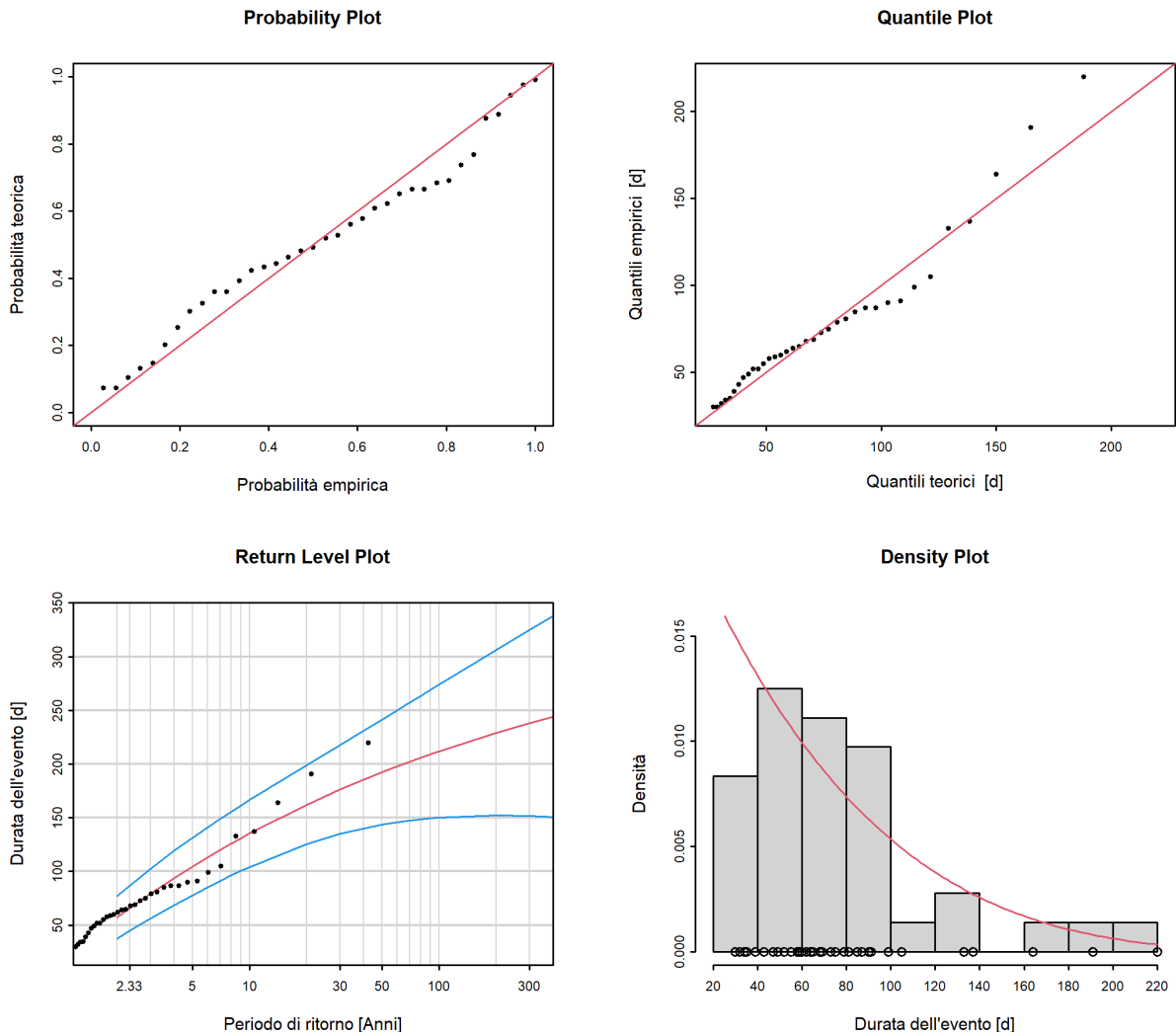
Figura 12: Plot diagnostici della variante di modello "stat" dell'approccio POT (01.06.1977 - 31.05.2019)
