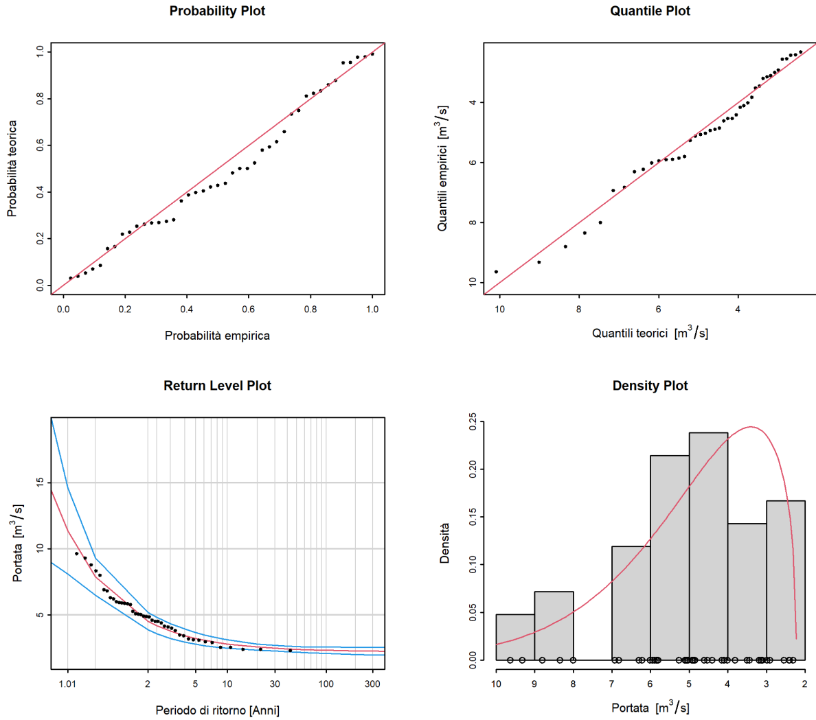
Figura 7: Plot diagnostici della variante di modello "stat" dell'approccio BLOCK (01.06.1977 - 31.05.2019)
