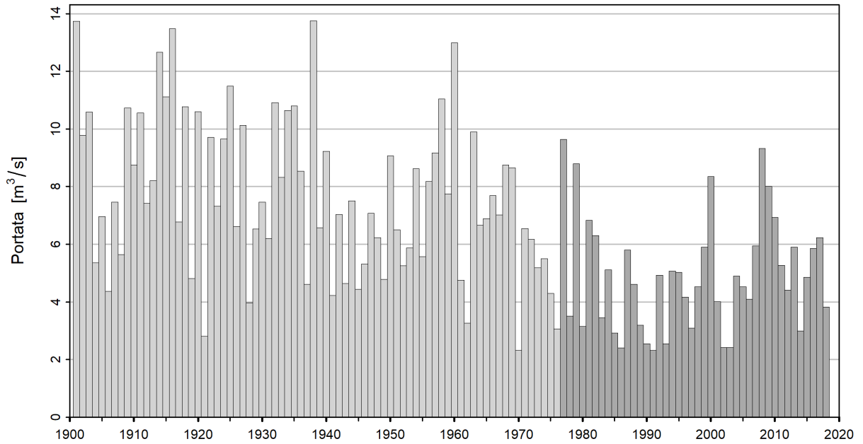
Figura 6: Serie temporale di NM7Q [ \text{m}^3/\text{s} ] (01.06.1901 - 31.05.2019), grigio chiaro: NM7Q non utilizzati, grigio scuro: NM7Q utilizzati
