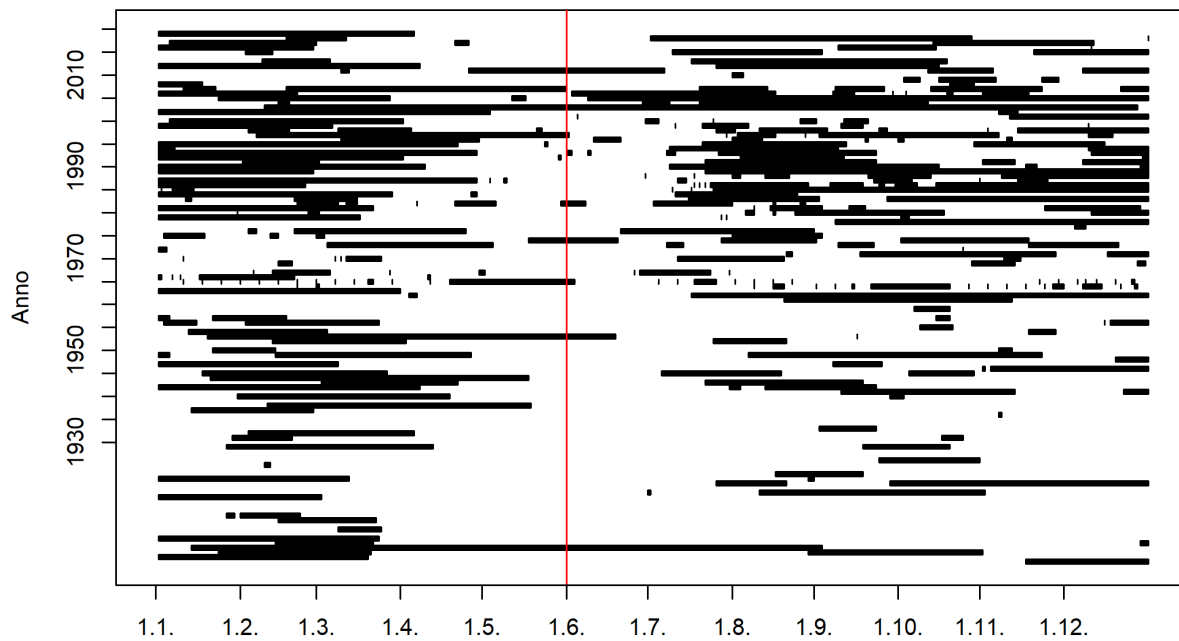
Figura 1: Apparizione temporale dei periodi di magra durante l'anno (01.06.1901 - 31.05.2019) e mese iniziale dell'anno di magra (linea rossa) 1
