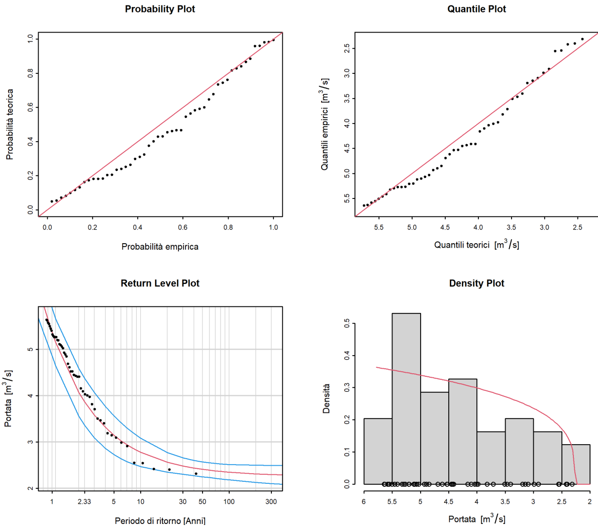
Figura 9: Plot diagnostici della variante di modello "stat" dell'approccio POT (01.06.1977 - 31.05.2019)
