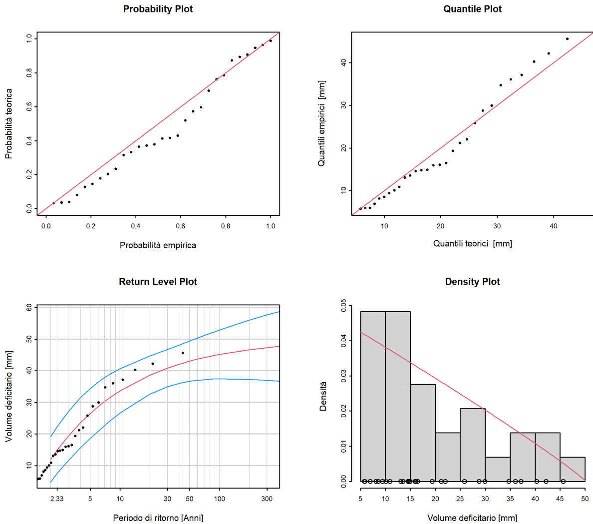
Figura 14: Plot diagnostici della variante di modello "stat" dell'approccio POT (01.06.1977 - 31.05.2019)
