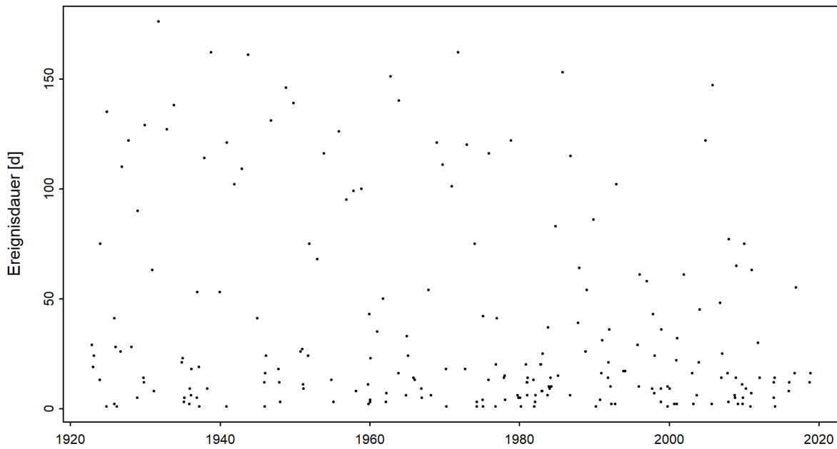
Abbildung 4: Zeitreihe der Niedrigwasserdauern [d] (01.06.1922 - 31.05.2019)
