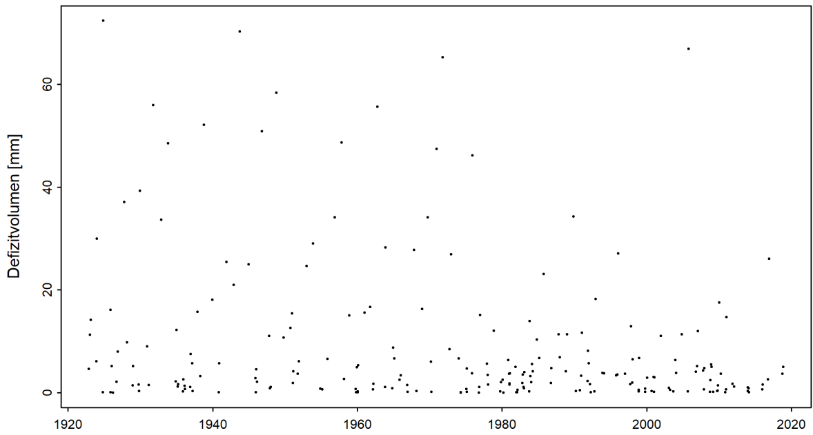
Abbildung 5: Zeitreihe der Defizitvolumen [mm] (01.06.1922 - 31.05.2019)
