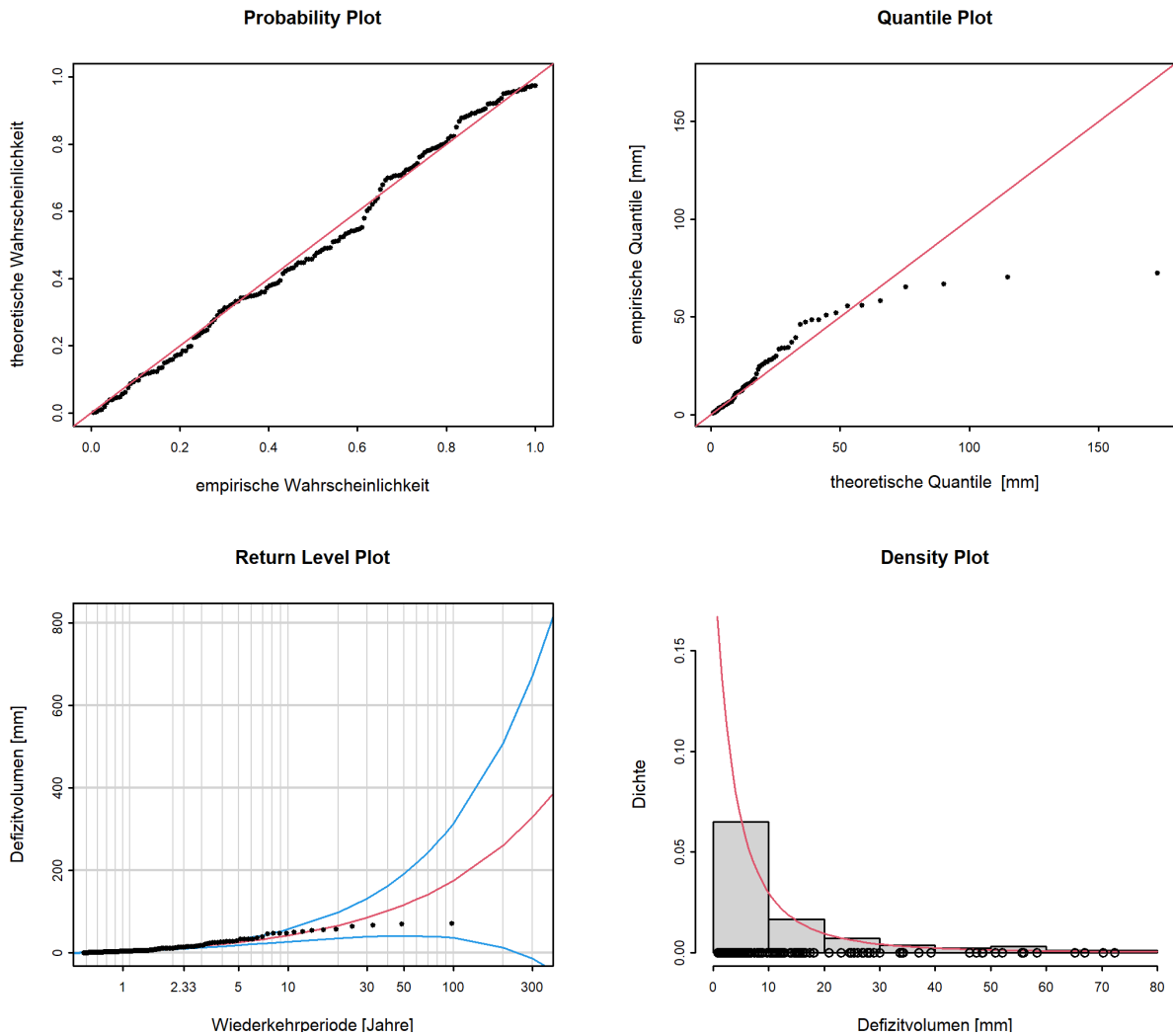
Abbildung 14: Diagnostikplots der Modellvariante “stat” des POT-Ansatzes (01.06.1922 - 31.05.2019)
