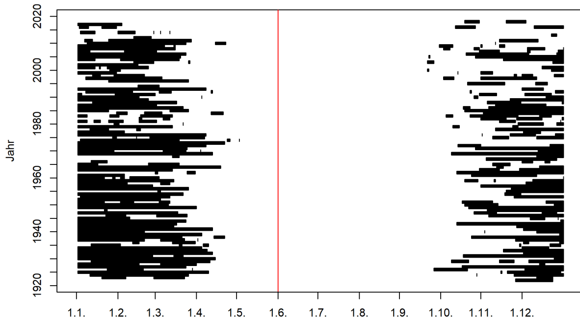
Abbildung 1: Zeitliches Auftreten der Niedrigwasserperioden im Jahresverlauf (01.06.1922 - 31.05.2019) und Startmonat des Niedrigwasserjahres (rote Linie) 1
