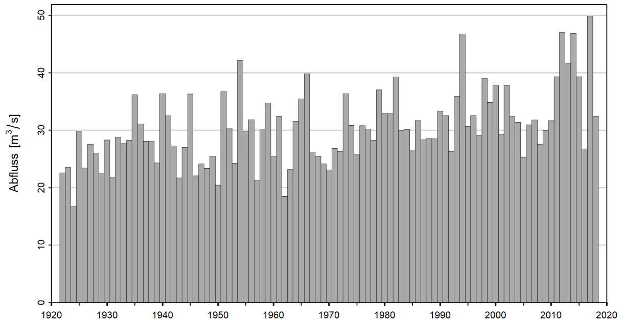
Abbildung 6: Zeitreihe der NM7Q [m³/s] (01.06.1922 - 31.05.2019)
