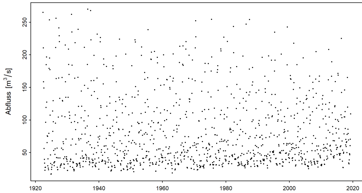
Abbildung 3: Zeitreihe der monatlichen Minima der M7Q [ \text{m}^3/\text{s} ] (01.06.1922 - 31.05.2019)
