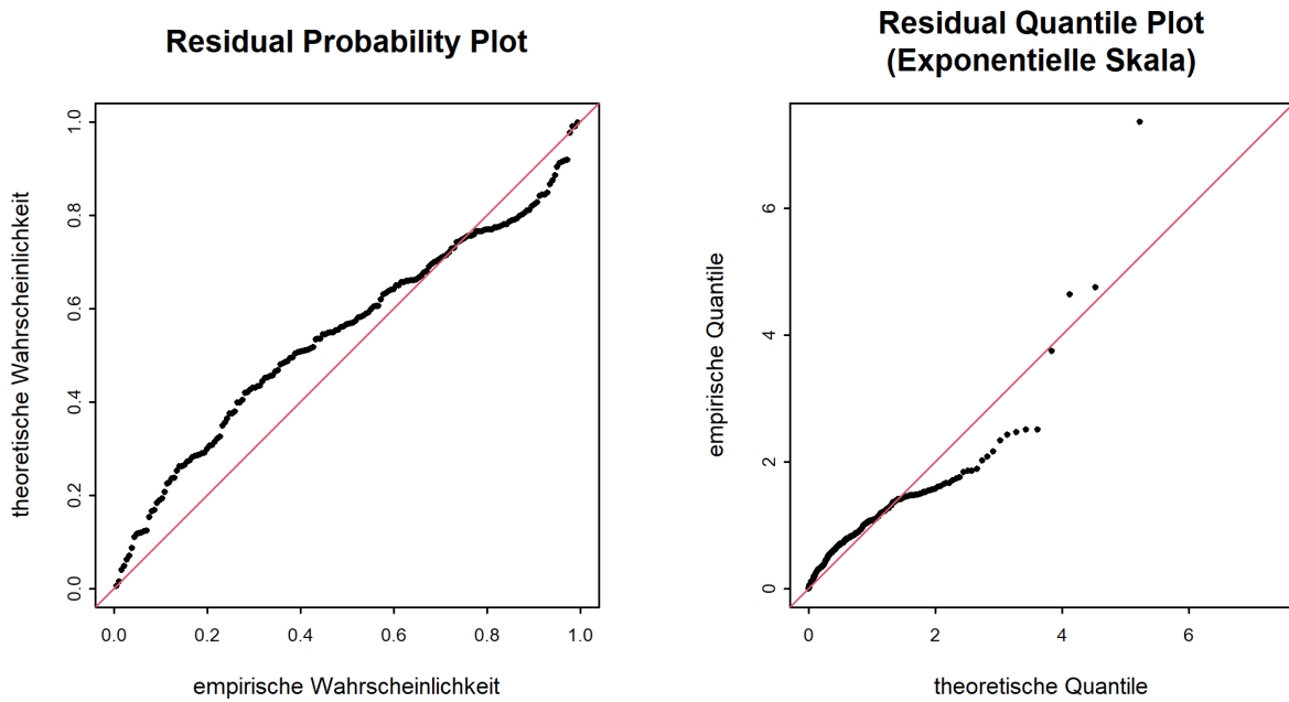
Abbildung 9: Diagnostikplots der Modellvariante "sigl" des POT-Ansatzes (01.06.1922 - 31.05.2019)
