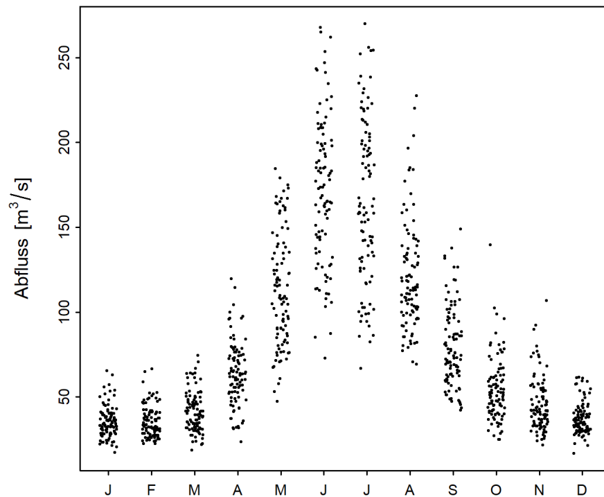
Abbildung 2: Saisonaler Verlauf der monatlichen Minima der M7Q [m³/s] (01.06.1922 - 31.05.2019)
