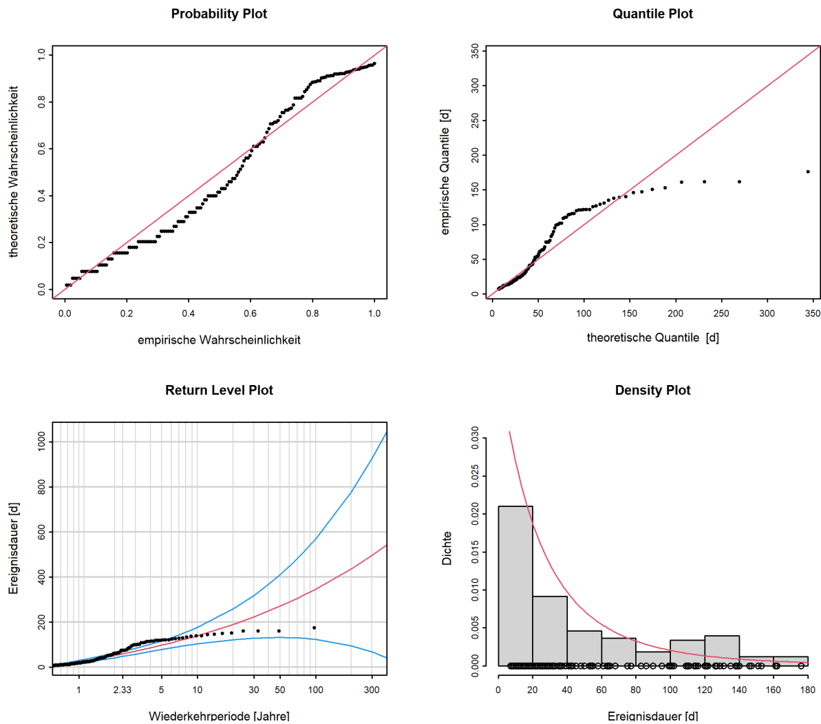
Abbildung 12: Diagnostikplots der Modellvariante “stat” des POT-Ansatzes (01.06.1922 - 31.05.2019)
