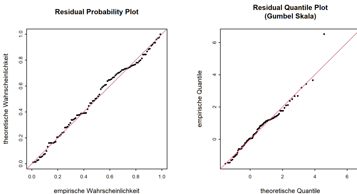
Abbildung 7: Diagnostikplots der Modellvariante "mul" des BLOCK-Ansatzes (01.06.1922 - 31.05.2019)
